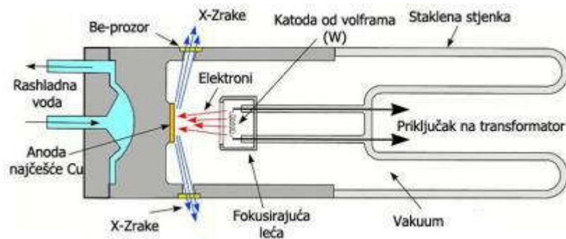
Slika 13. Shematski prikaz rentgenske cijevi [18]
