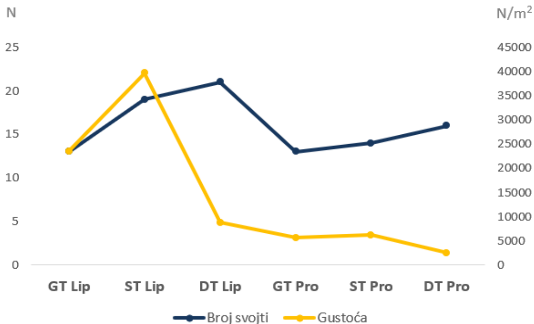
Slika 10. Gustoća zajednice makrozoobentosa izražena kao broj jedinki po jediničnoj površini ( 1 \text{ m}^2 ) i broj svojti unutar zajednice makrozoobentosa na tri postaje duž rijeke Krčiča (GT – gornji tok, ST – srednji tok, DT – donji tok) u različitim sezonama uzorkovanja (Lip – lipanj, Pro – prosinac).
