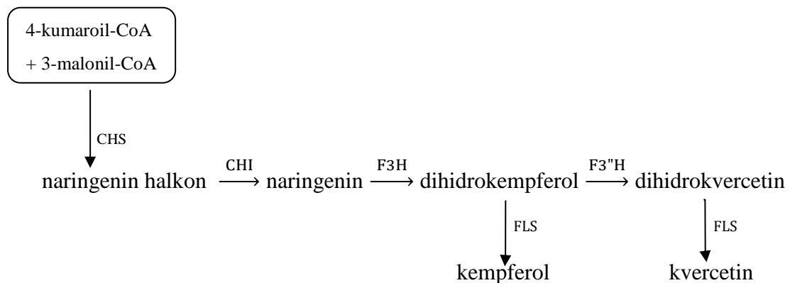
Slika 6. Biosintetski put flavonoida; CHS = halkon-sintaza, CHI = halkon-izomeraza, F3H = flavanon-3-hidroksilaza, F3'H = flavonoid-3'-hidroksilaza, FLS = flavonol-sintaza (preuzeto i prilagođeno iz izvora Falcone Ferreyra i sur. 2012).
