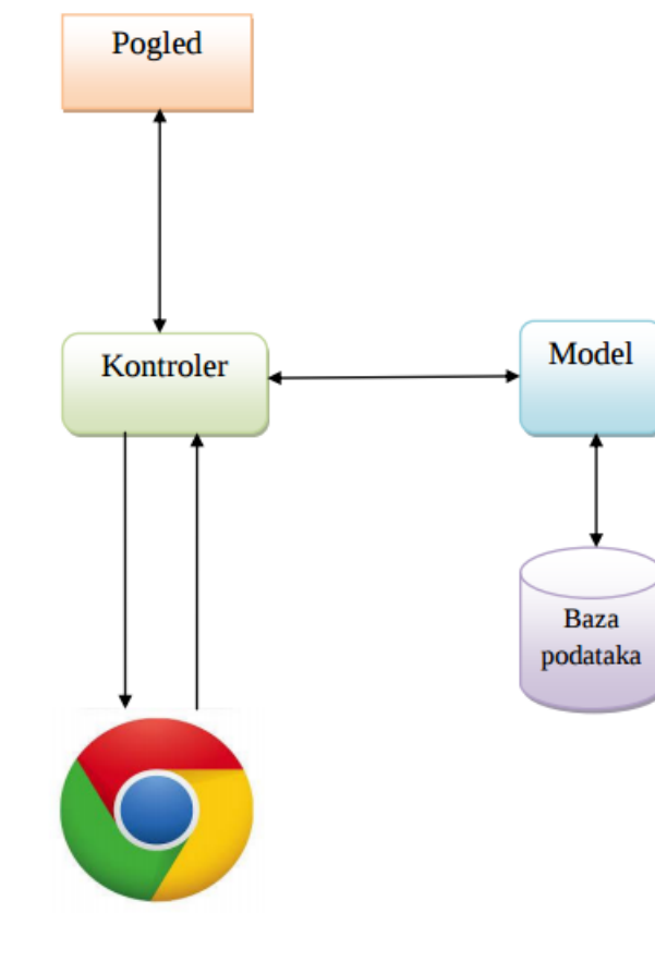
Slika 2.3: Shematski prikaz principa rada MVC arhitekture
