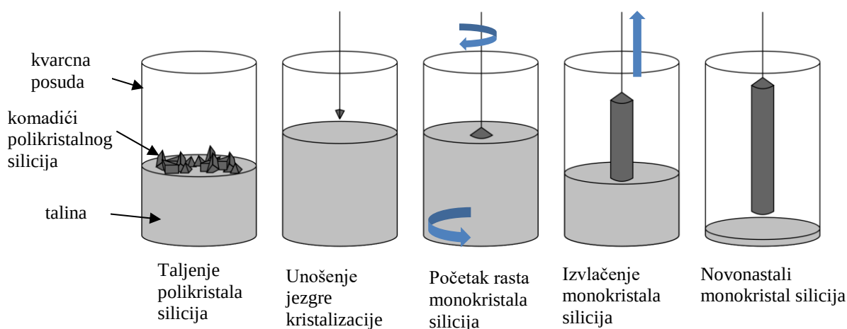
Slika 15. Shematski prikaz dobivanja monokristala silicija Czoehrlskijevim procesom.
