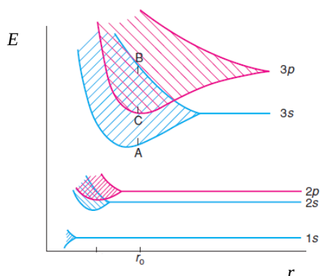
Slika 4. Efekt udaljenosti između susjednih atoma natrija na energetska stanja i vrpce natrija.
