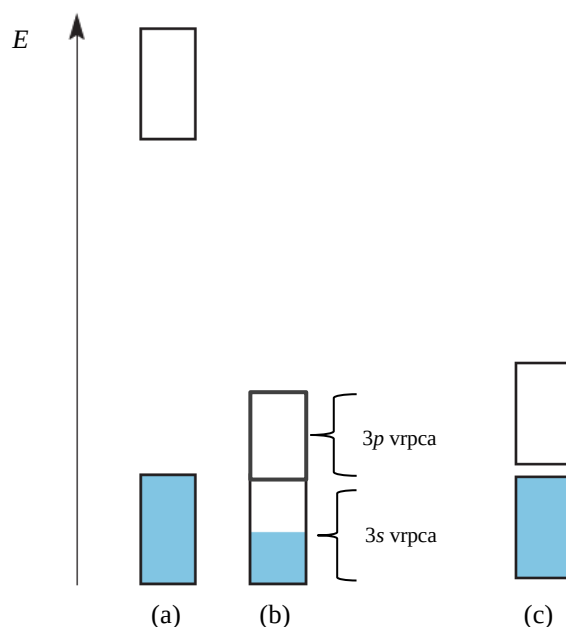
Slika 3. Struktura vrpce a) izolatora, b) vodiča i c) poluvodiča. Plavom bojom prikazana su popunjena energetska stanja, a bijelom prazna. Preuzeto iz ref. 1 i dorađeno.
