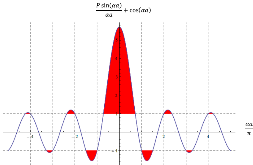
Slika 7. Ovisnost E(k) prikazana preko ovisnosti
