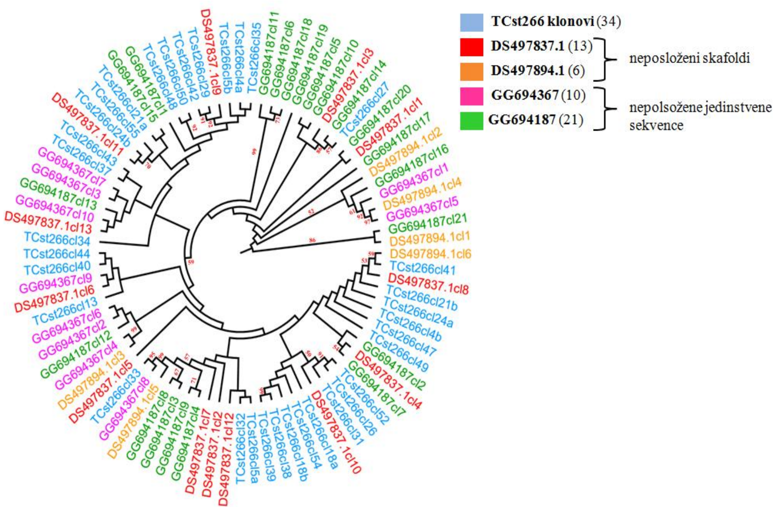
Slika 7. Filogenetski odnosi monomera satDNA TCst266 vrste Tribolium castaneum dobiveni metodom najveće vjerojatnosti prema Tamura-3-parametarskom modelu uz dodatak gamma distribucije (T92+G). Brojevi na granama predstavljaju postotak stabala koja su podržala prikazanu topologiju u nasumičnoj statističkoj analizi u 500 navrata (prikazane su samo bootstrap podrške koje prelaze 50%). Popratnom legendom objašnjeno je porijeklo monomera. Monomeri označeni s TCst266 predstavljaju in silico ekstrahirane monomere iz
