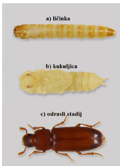
Slika 2. Različiti životni stadiji kukca Tribolium castaneum (preuzeto i modificirano iz Khan i sur. 2016).
