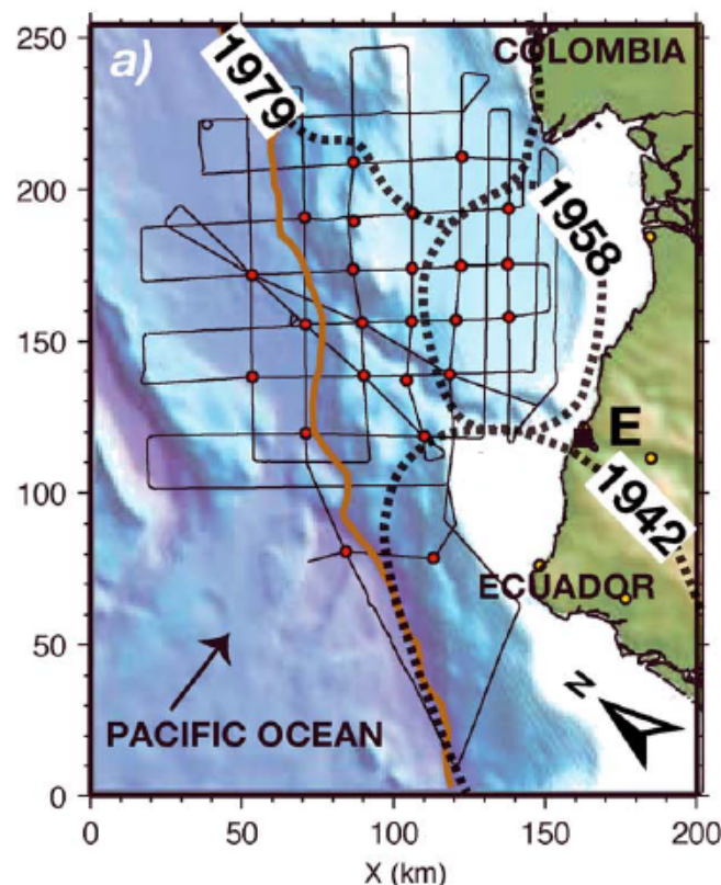
Slika 3.2: Dio lokalnog koordinatnog sustava. Tanke linije su linije ispaljivanja, crveni kružići su OBS-ovi. Debeli smeđa linija prikazuje oceanski jarak. Isprekidanim linijama označena su područja loma potresa iz 1942., 1958. i 1979. Crni kvadrat (E) označava grad Esmeraldas. Crna strelica pokazuje smjer konvergencije oceanske ploče. Preuzeto iz García-Cano i sur. [2014].
