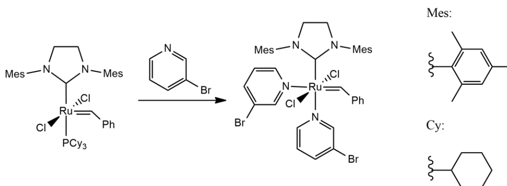
Slika 9. Sinteza Grubbsova katalizatora treće generacije. 6
