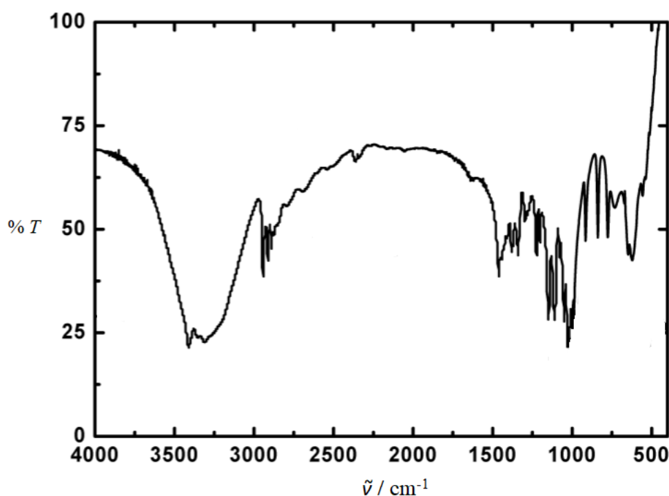
Slika 2.9. FT-IR spektar \alpha -D-glukoze. 7
