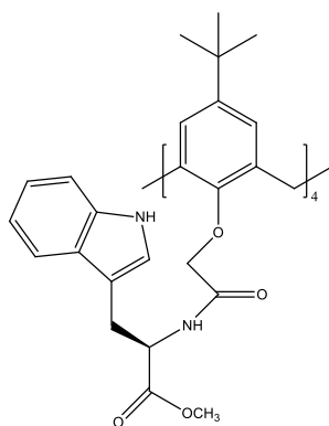
Slika 29. Struktura peptidokaliks[4]arena. 9
