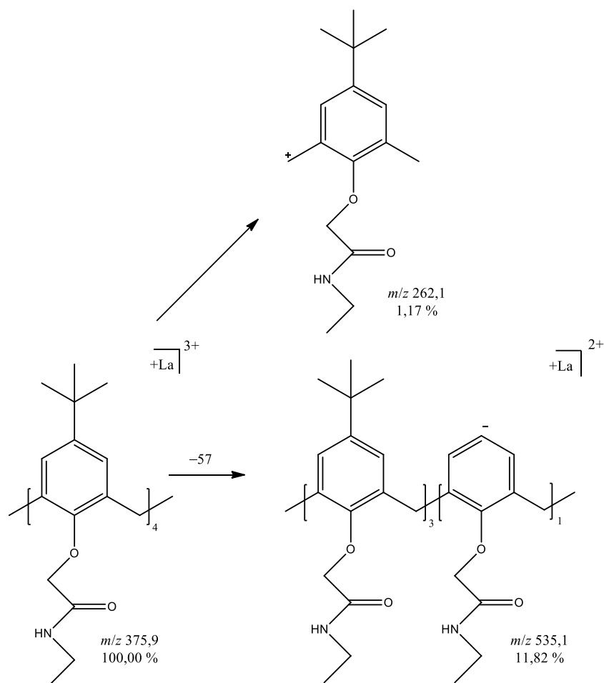
Slika 42. Shema fragmentiranja kompleksnog iona spoja 2 i \text{La}^{3+} ( [\text{M}+\text{La}]^{3+} , m/z = 375,9 ).
