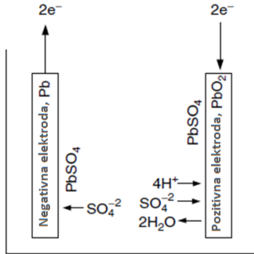
Slika 7: Pražnjenje olovno - kiseline baterije [2]
