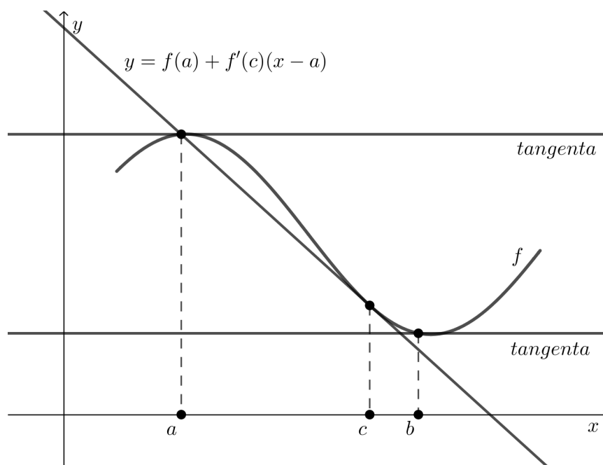
Slika 1.4: Geometrijska interpretacija Flettovog teorema
