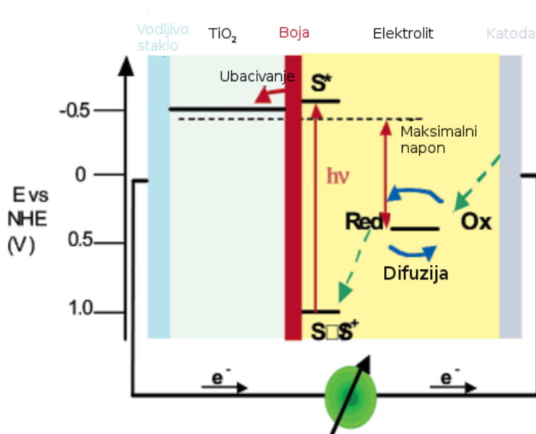
Slika 2.1: Shema DSSC [6].
