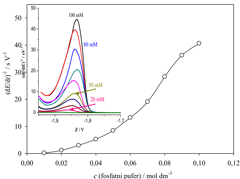
Slika 13. AdT CPS ovisnost visine pika kitozana ( c = 50 \times 10^{-6} g cm^{-3} ) u fosfatnom puferu, pH 7,05 koncentracija od 0,01 mol dm^{-3} do 0,1 mol dm^{-3} ; E_a = -0,1 V , t_a = 60 s , I_{str} = -20 \mu A .
