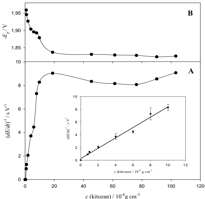
Slika 16. Ovisnost visine (A) i položaja (B) pika H_{PS} kitozana s povećanjem koncentracije kitozana u fosfatnom puferu pH 7,05. Uvjeti mjerenja: E_a = -0,1 V, I_{str} = -20 \mu A, t_a = 60 s
