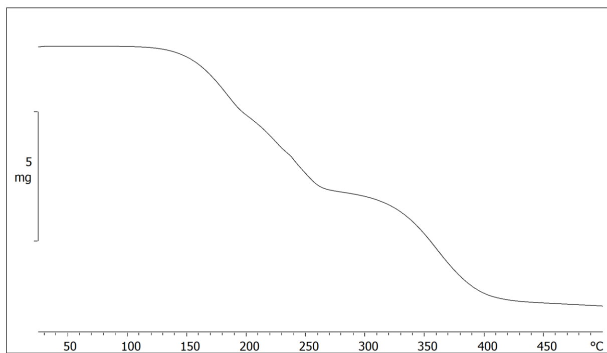
Slika D23. TG krivulja kokristala (\text{CHI}_3)_3(\text{N-Me-CIPyI})_2 .
