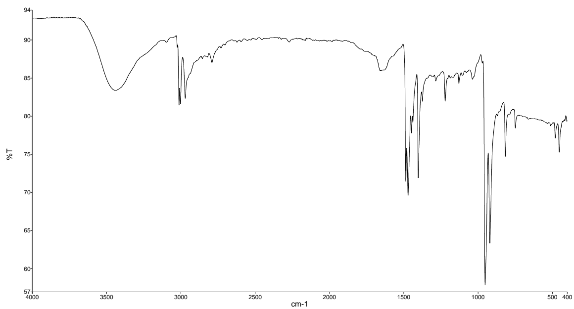
Slika D47. IR spektar ionskog spoja DiMeTemedI 2 .
