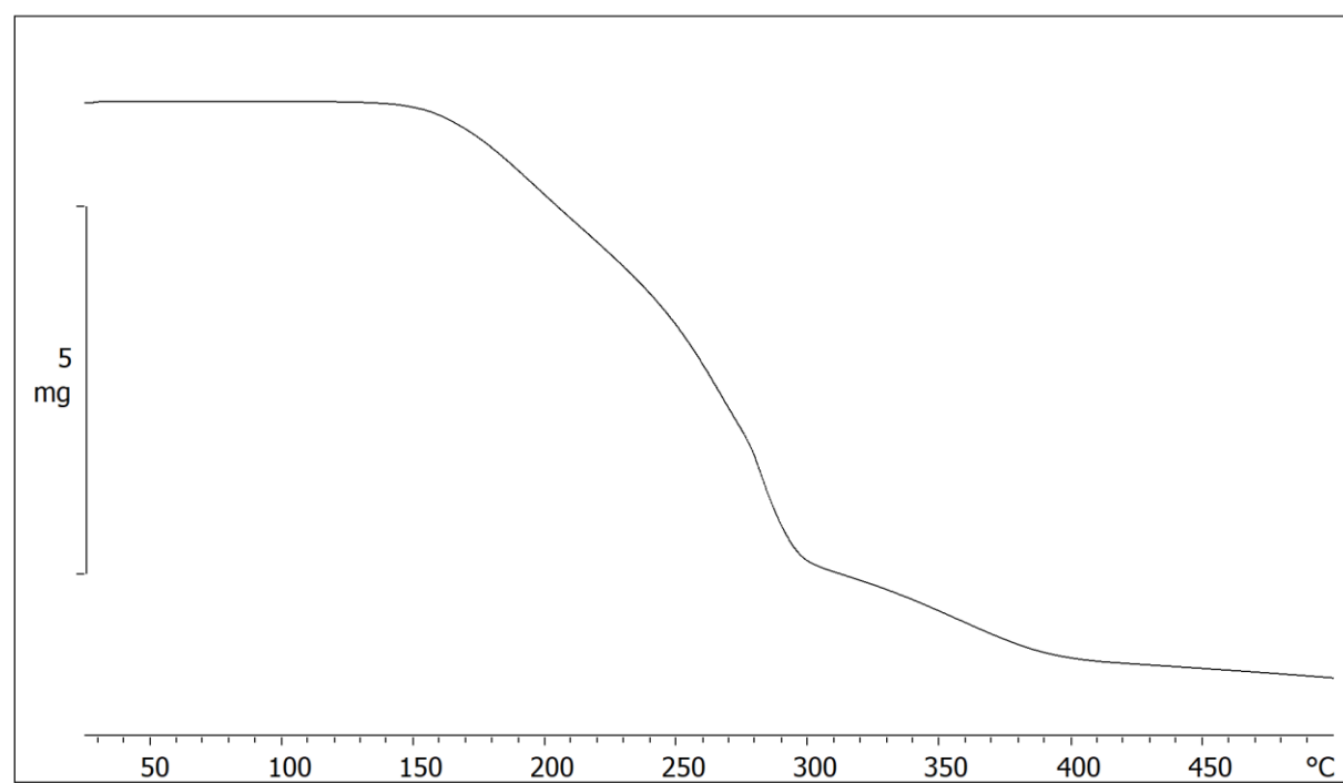
Slika D29. TG krivulja kokristala (\text{CHI}_3)(\text{N-Me-3-IPyI}) .
