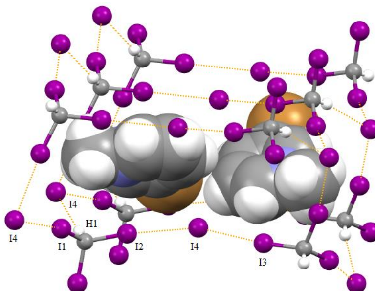
Slika 22. Prikaz anionske mreže kokristala (CHI 3 )(N-Me-3-BrPyI). Kation N-Me-3-BrPy + prikazan je kalotnim modelom, atomi i veze anionske mreže prikazani su stilom štapića i kuglica.
