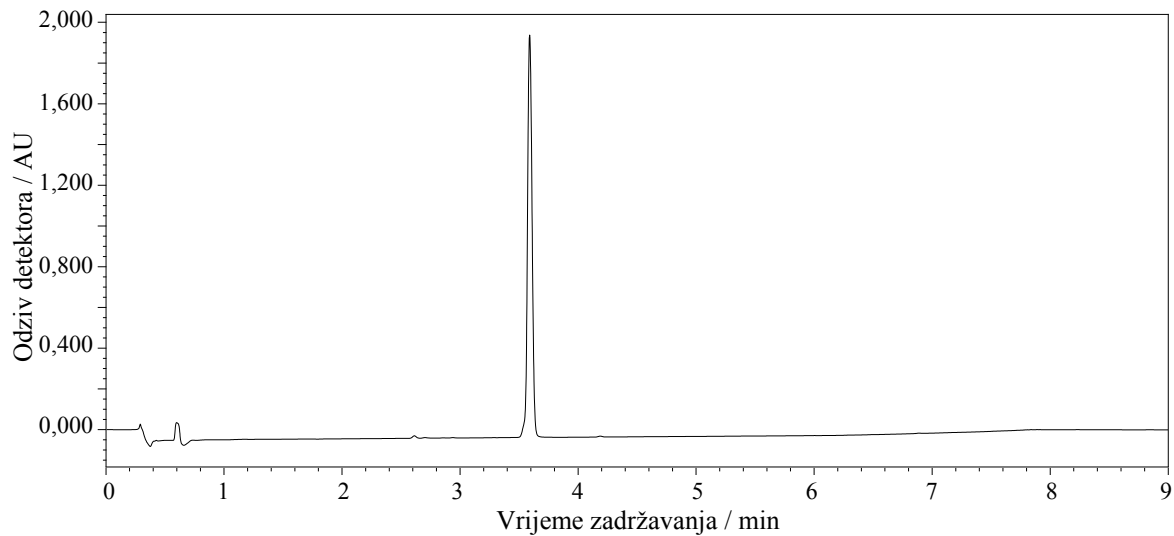
Slika 88. UHPLC-UV-DAD kromatogram spoja 6 izoliranog iz uzorka II 3-brom-5-(trifluormetil)anilina pri 224 nm.
