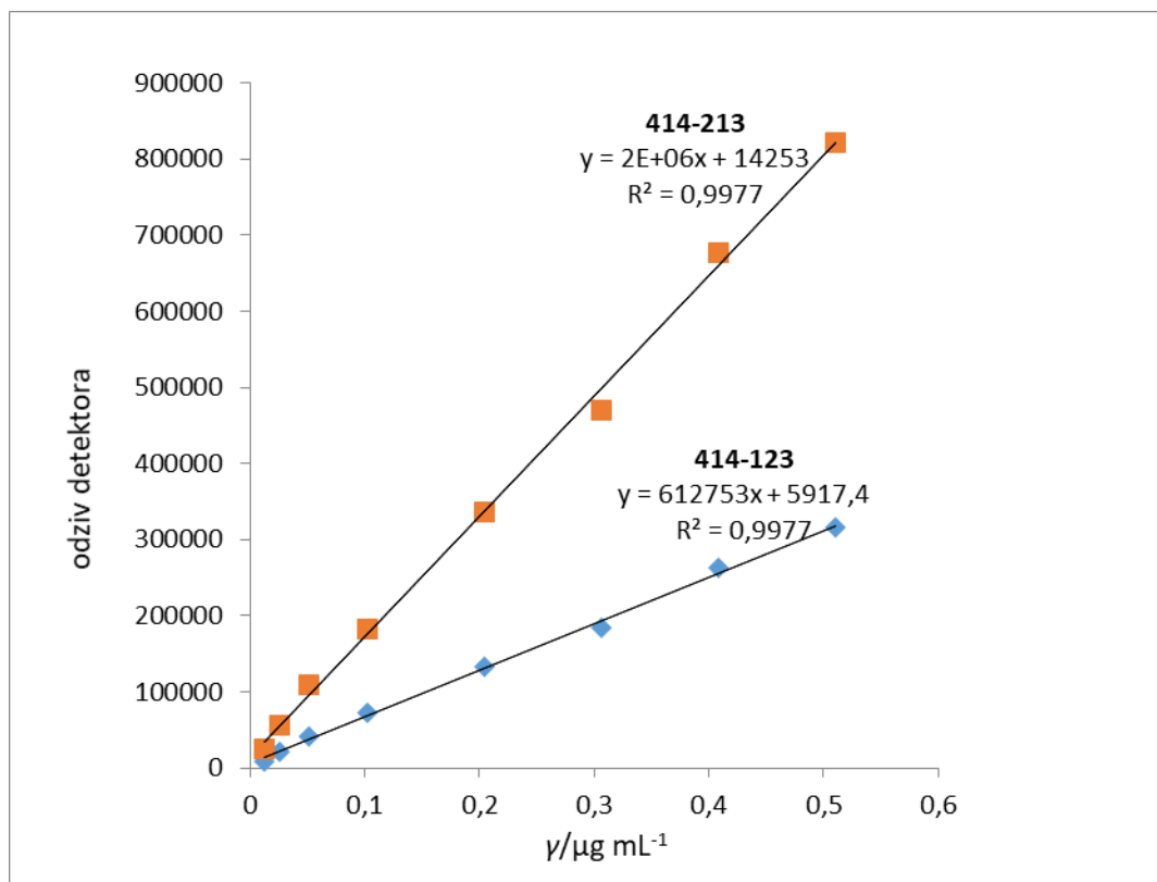
Slika 27. Kalibracijski pravci za modelne otopine benzaldehid-Z-Glu-OEt-hidrazida ( 7a ) s dva MRM prijelaza: kvantifikacijski 414-213 i potvrđni 414-123
