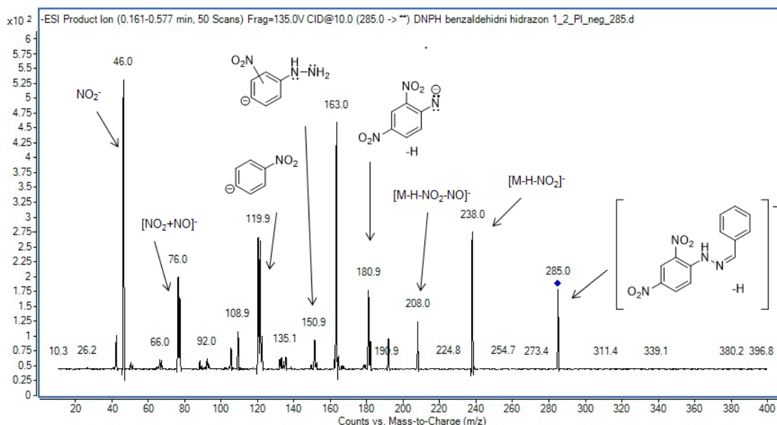
Slika 20. MS/MS spektar molekulskog iona [M-H]^- m/z 285 benzaldehid-2,4-DNP-hidrazona (6a)
