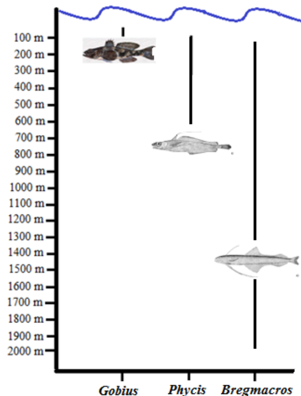
Slika 34. Rasponi dubina na kojima žive nađeni rodovi riba na lokalitetu Veternica
