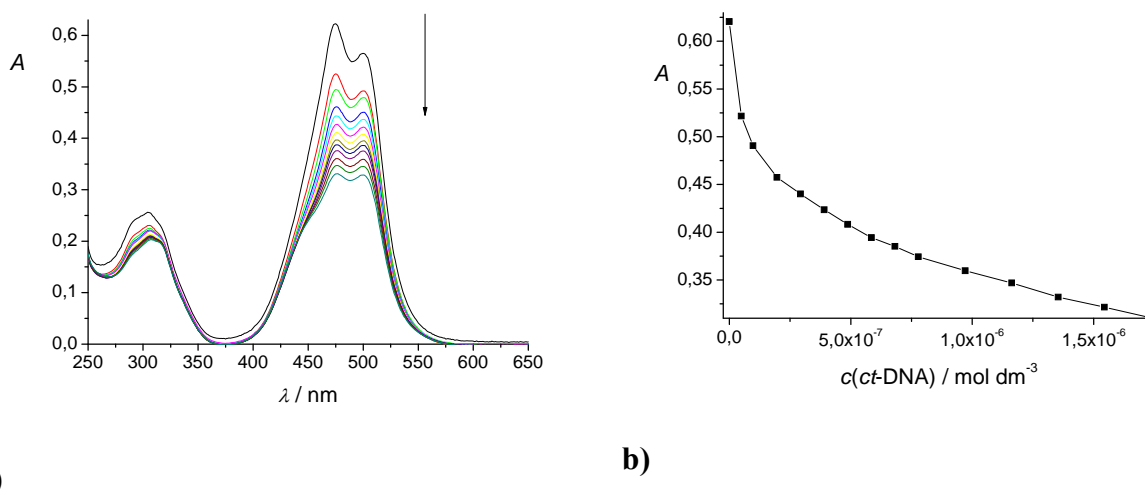
Slika 17. a) UV/Vis titracija 6-Cl-TO-1 ( c = 1,76 \times 10^{-5} \text{ mol dm}^{-3} ) s ct -DNA; b) Promjene u UV/Vis spektru 6-Cl-TO-1 pri \lambda_{\text{max}} = 473 \text{ nm} kao posljedica titracije s ct -DNA, u kakodilatnom puferu, \text{pH} = 7 , I = 0,05 \text{ mol dm}^{-3} pri 25 \text{ }^\circ\text{C} .
