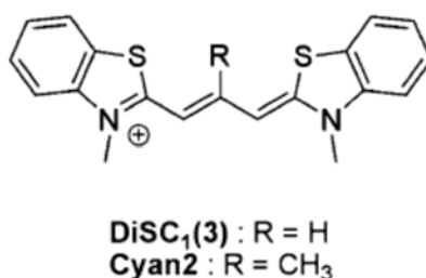
Slika 28: Molekulske strukture analoga simetričnih cijaninskih boja DiSC 14
