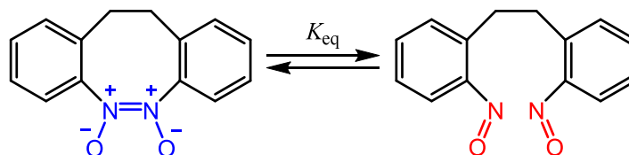
Slika 17. Primjer ravnoteže između zatvorenog azodioksidnog i otvorenog nitrozo oblika aromatskog dinitrozo spoja.
