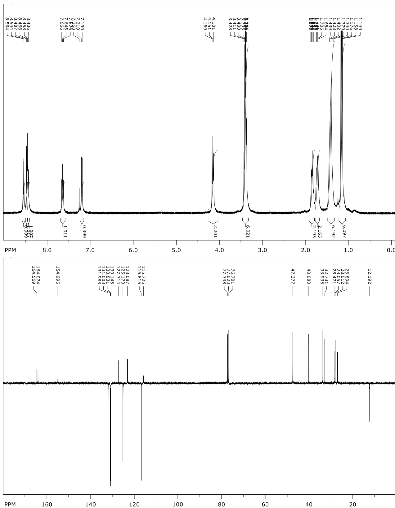
Prilog 68. Spektri ^1\text{H} NMR ( \text{CDCl}_3 , 400 MHz) i ^{13}\text{C} NMR ( \text{CDCl}_3 , 100 MHz) spoja 70
