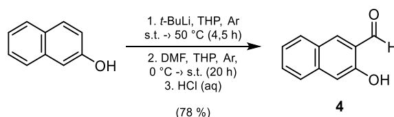
Shema 74. Priprava karbaldehida 4 u jednom koraku 296
