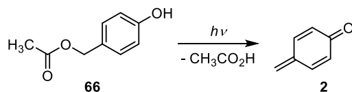
Shema 22. Fotoeliminacija octene kiseline iz derivata fenola 66 uz nastanak p -QM ( 2 ) 96
