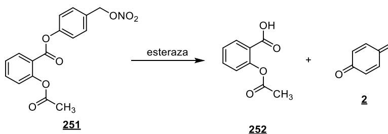
Shema 60. Metabolička aktivacija NO-aspirina ( 251 ) 115
