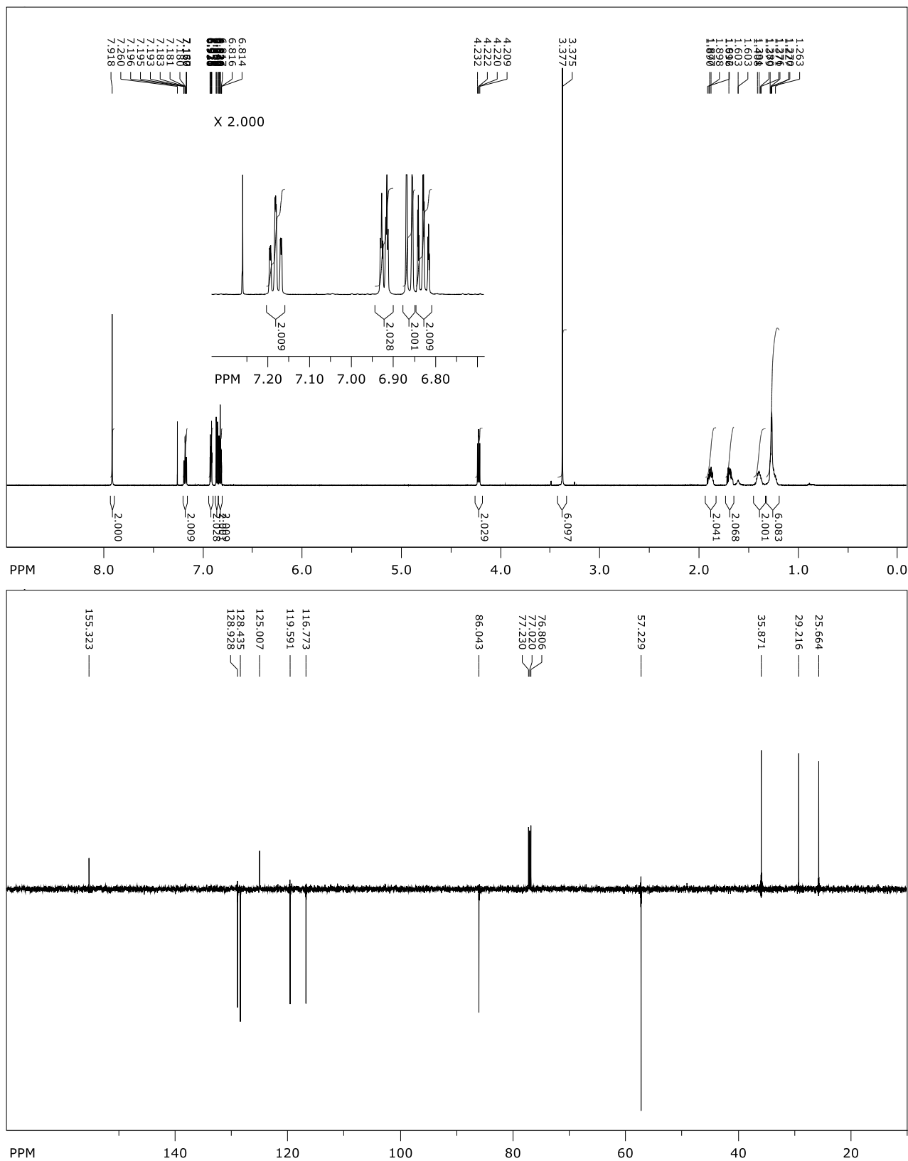
Prilog 25. Spektri ^1\text{H} NMR ( \text{CDCl}_3 , 600 MHz) i ^{13}\text{C} NMR ( \text{CDCl}_3 , 150 MHz) spoja 24
