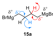
Slika 46. Struktura i prikaz reaktivnih \beta -H atoma u di-Grignardovom reagensu 15a
