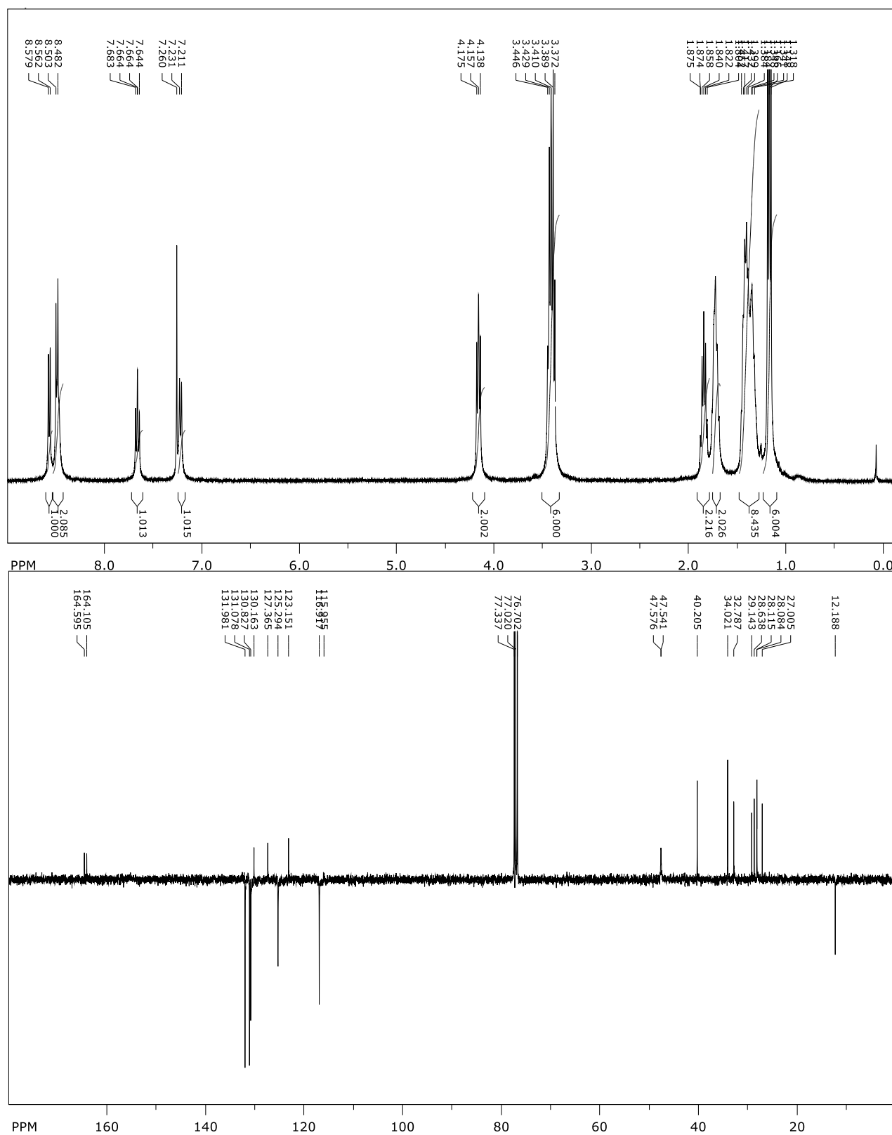
Prilog 69. Spektri ^1\text{H} NMR ( \text{CDCl}_3 , 400 MHz) i ^{13}\text{C} NMR ( \text{CDCl}_3 , 100 MHz) spoja 71
