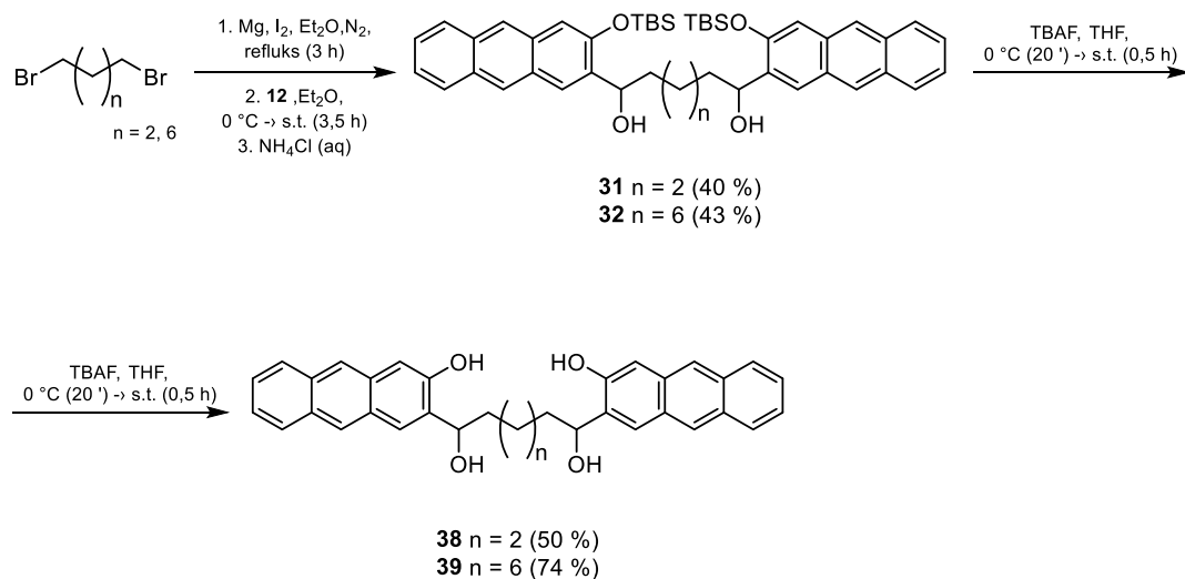
Schema 81. Priprema antrolnih homobifunkcionalnih spojeva
