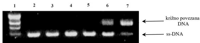
Slika 19. Elektroferogram linearizirane plazmidne DNA (pBR322) (0,7 \mu\text{g} ) pri različitim koncentracijama spoja 204 ( 3 – 50 \mu\text{M} , 5 – 0,1 \mu\text{M} , 6 – 1 \mu\text{M} , 7 – 10 \mu\text{M} ) u fosfatnom puferu (pH = 7,7). Smjese DNA i spoja 204 osvijetljene su na 400 nm kroz 30 min (jažice 5 , 6 i 7 ) i razdvojene alkalnom agaroznom gel-elektroforezom. Lambda HindIII DNA (jažica 1 ) korišten je kao standard molekulske mase. U jažici 2 nalazi se DNA koja nije tretirana spojem 204 , u jažici 3 nalazi se DNA tretirana spojem 204 ali bez osvijetljavanja, a u jažici 4 nalazi se osvijetljena (30 min, 400 nm) DNA 147
