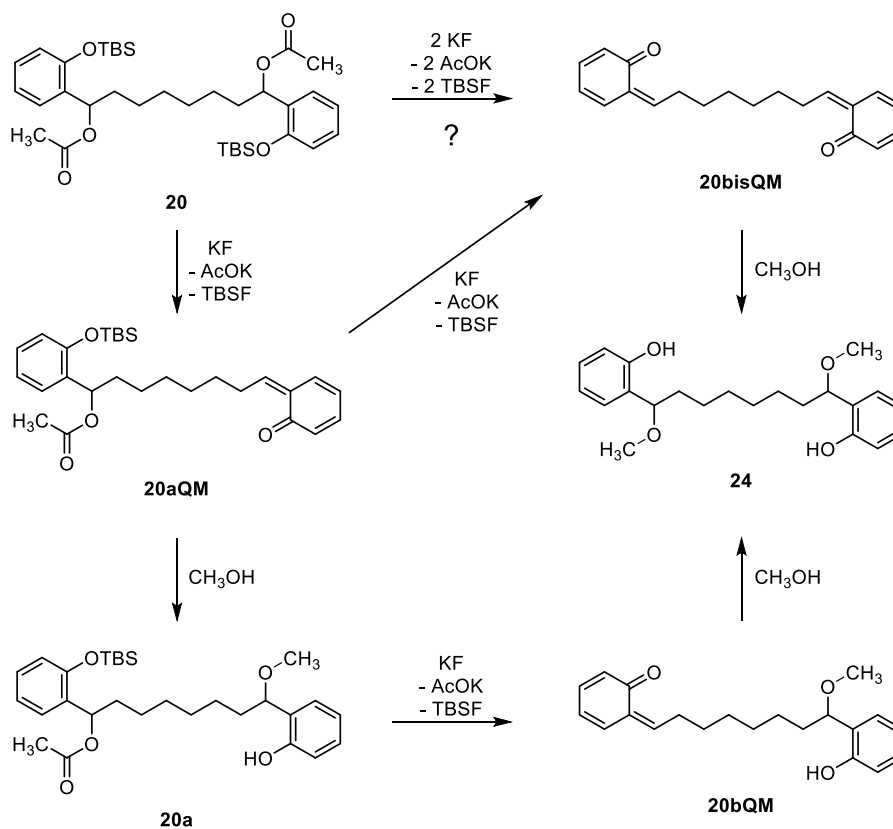
Shema 84. Mogući putevi reakcija nastanka i hidrolize QM iz spoja 20
