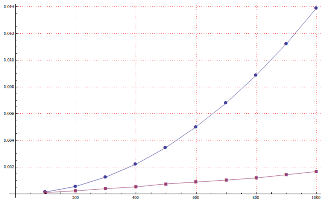
Slika 3.1: ● brute_force; ■ Divide_and_Conquer
