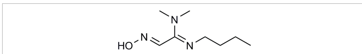
Slika 2.20. Vodeći amidin-oksinski reaktivator N-[2-(butyliminoil)-2-(dimetilamin)etiliden]hidroksilamin. 163
