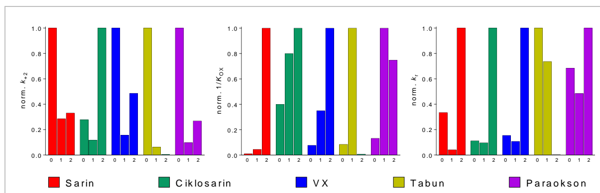
Slika 4.15. Ovisnost maksimalne konstante brzine reaktivacije ( k_{+2} ), afiniteta inhiranog enzima prema oksimu ( 1/K_{OX} ) i ukupne konstante brzine reaktivacije ( k_r ) za reaktivaciju AChE inhirane sarinom, ciklosarinom, VX-om, tabunom ili paraoksonom o broju atoma klora vezanih na piridinijev prsten s oksimskom skupinom (naznačeno na apscisi: 0 za oksim K027, 1 za oksim K865 i 2 za oksim K868).
