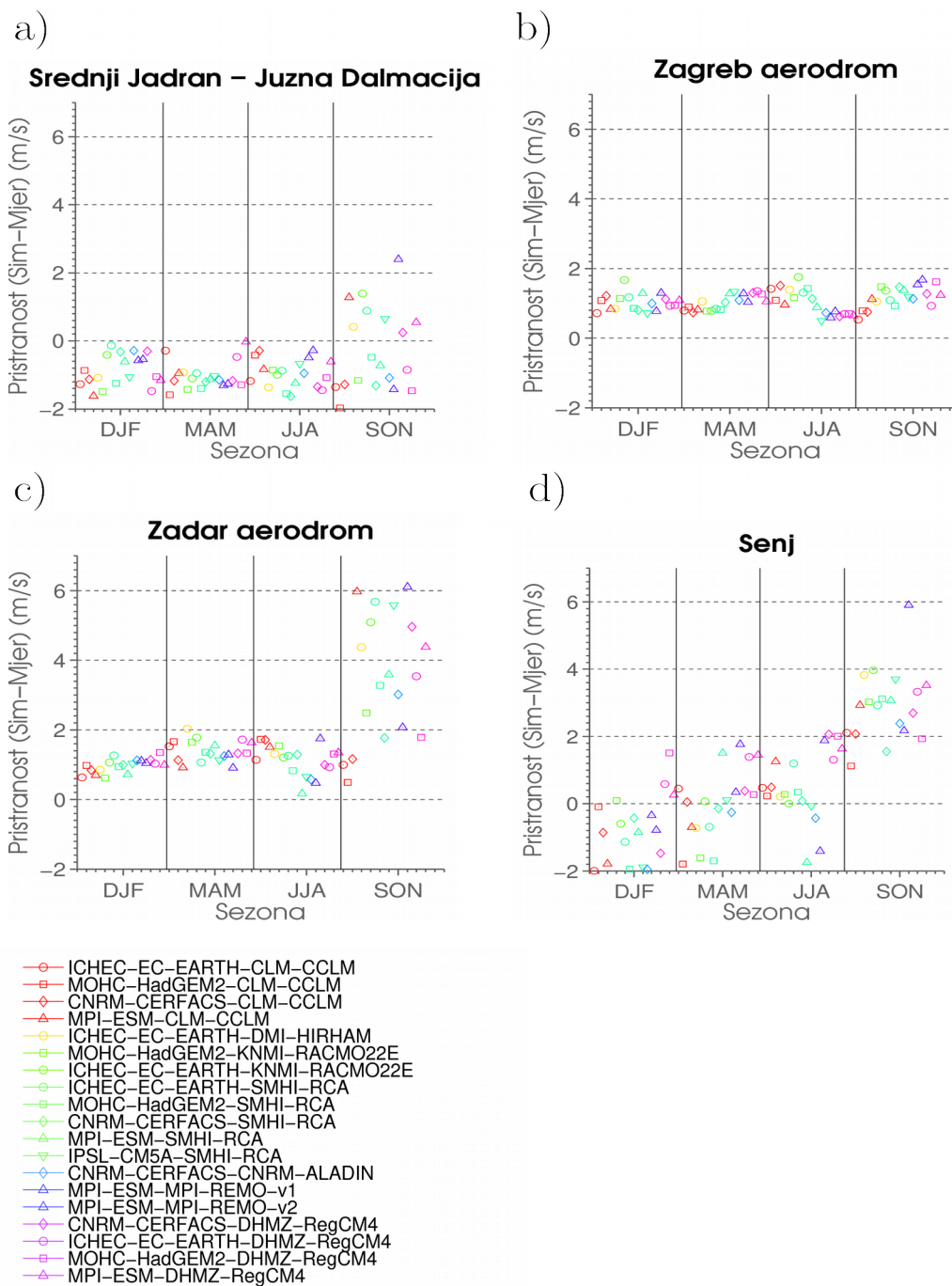
Slika 22. Pristranost brzine vjetrova za: a) Srednji Jadran - Južna Dalmacija, b) zračnu luku Zagreb, c) zračnu luku Zadar, d) Senj za razdoblje 2001.-2005. godine. Boje označavaju pojedinu simulaciju, dok simbol označava pojedini GCM kao što je naznačeno legendom.
