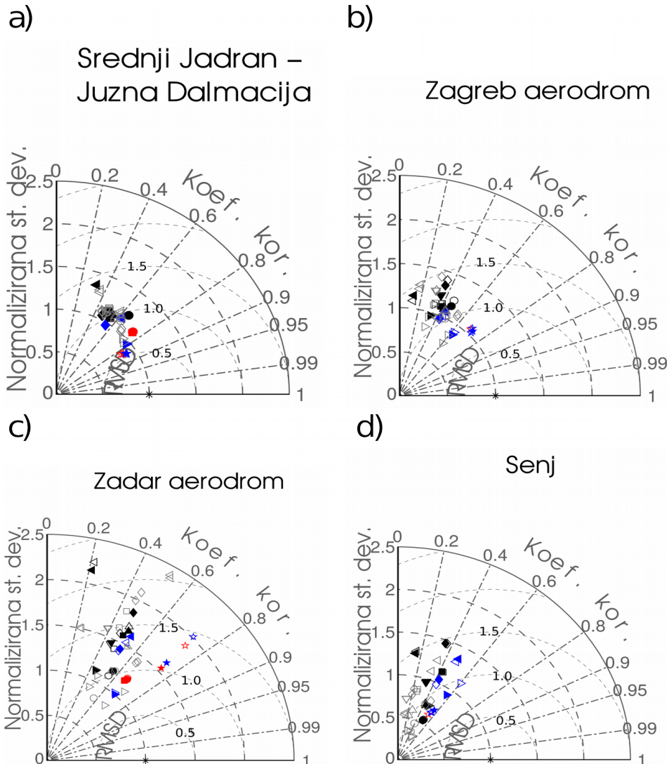
Slika 7. Normalizirani Taylorov dijagram brzine vjeta prikazuje uspješnost simulacija obzirom na mjerene vrijednosti za: a) lokaciju nad otvorenim morem (Srednji Jadran - Južna Dalmacija, 2001.-2008.), b) postaju u unutrašnjosti (zračna luka Zagreb, 1996.-2008.), c) obalnu postaju u ravničarskom terenu (zračna luka Zadar, 2001.-2008.) i d) obalnu postaju u kompleksnom terenu (Senj, 1996.-2008.). Prazni simboli označavaju NN metodu interpolacije, a puni simboli BI metodu interpolacije, crni simboli označavaju EURO-CORDEX-11 simulacije, plavi MED-CORDEX simulacije, crveni ETHZ simulacije, zvijezdice označavaju ERA-Interim simulacije, sivi simboli CORDEX-44 simulacije. Crna zvijezdica na x-osi predstavlja mjerenja.
