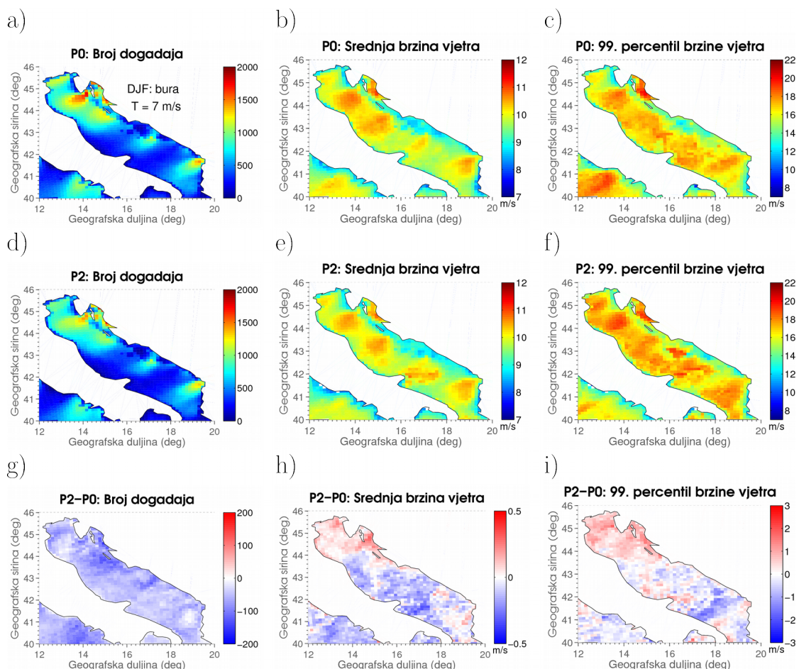
Slika 32. Rezultati za buru ( 22.5^{\circ} - 67.5^{\circ} ) u zimskoj (DJF) sezoni prikazani kao medijan ansambla od devet RCM simulacija u (a-c) medijan za P0 , (d-f) medijan za P2 i (g-i) medijan razlika 30-ogodišnjih razdoblja P2-P0 za pojedinačne simulacije. (a, d, g) broj događaja, (b, e, h) srednja brzina vjetra, (c, f, i) 99. percentil brzine vjetra. Prag brzine je 7 m/s, a scenarij je RCP8.5.
