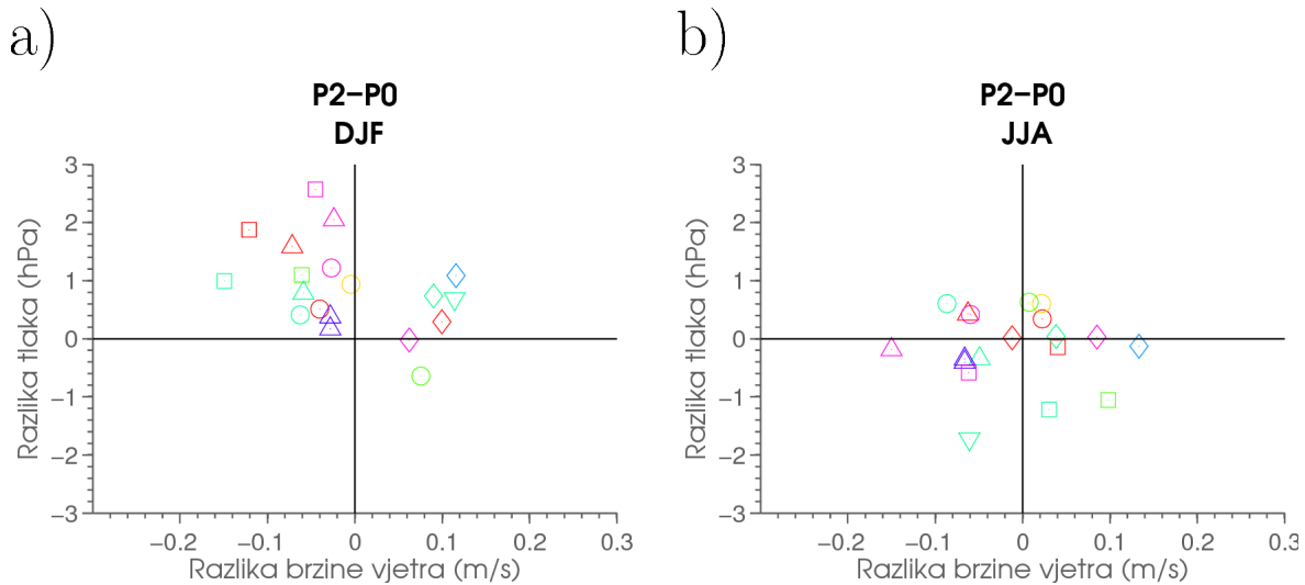
Slika 26. Promjene u polju prizemnog tlaka ( y - os) i vjetra ( x - os) u zimskoj (DJF) i ljetnoj (JJA) sezoni za RCP8.5 scenarij u P2 razdoblju u odnosu na P0 za sve dostupne simulacije nad morem jadranske domene (bijeli kvadrat na Sl. 21-23). Svaki GCM prikazan je jednim simbolom, a svaki RCM jednom bojom kao na Slici 22.
