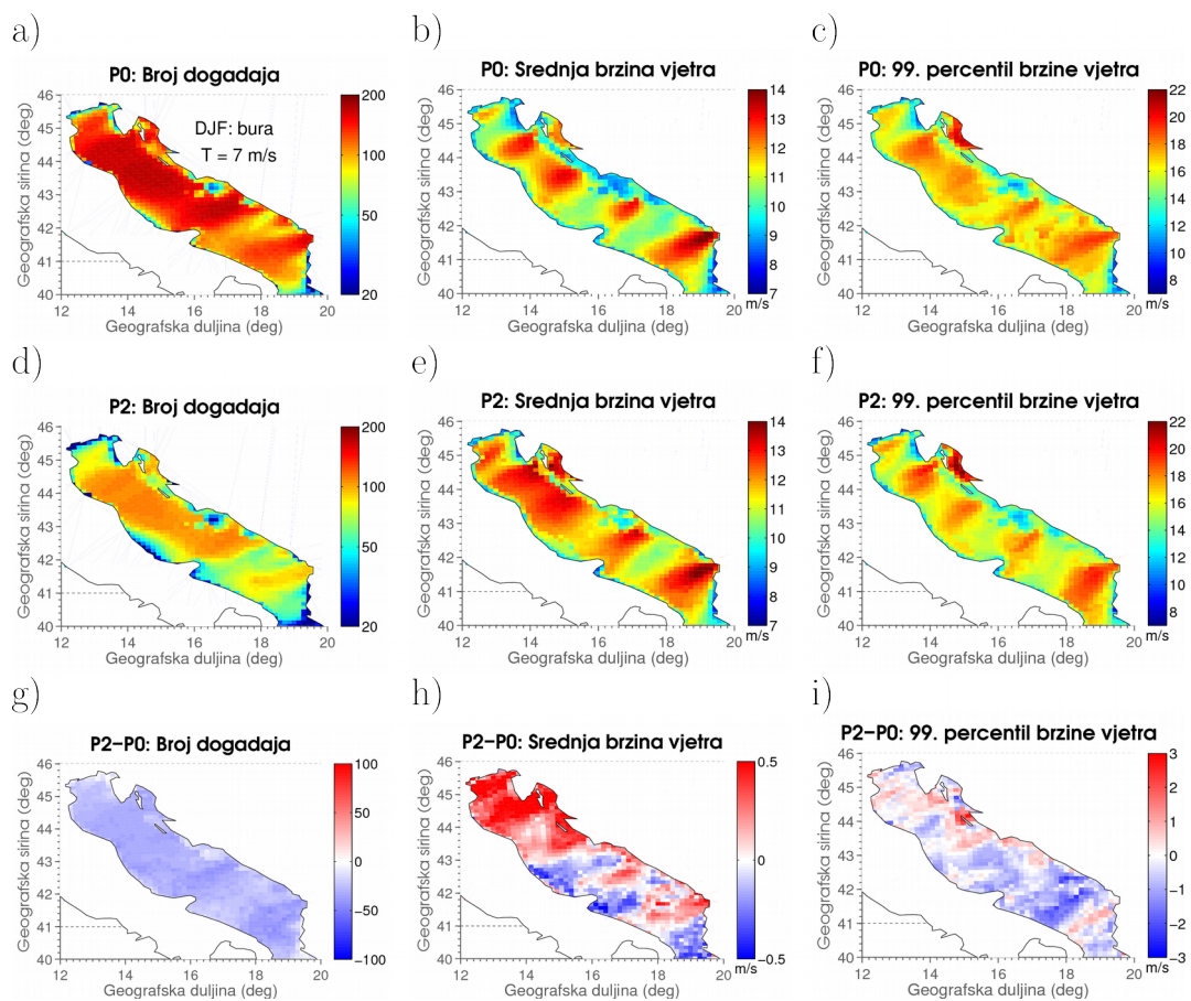
Slika C1. Rezultati za buru ( 22.5^{\circ} - 67.5^{\circ} ) u zimskoj (DJF) sezoni prikazani kao medijan ansambla od devet RCM simulacija u (a-c) medijan za P_0 , (d-f) medijan za P_2 i (g-i) medijan razlika P_2-P_0 za pojedinačne simulacije. (a, d, g) broj događaja, (b, e, h) srednja brzina vjetra, (c, f, i) 99. percentil brzine vjetra. Prag brzine je 7 m/s, a dodan je uvjet da barem 50% točaka preko Jadrana mora zadovoljavati uvijek za raspon kutova i brzinu. Scenarij koncentracije stakleničkih plinova je RCP8.5.
