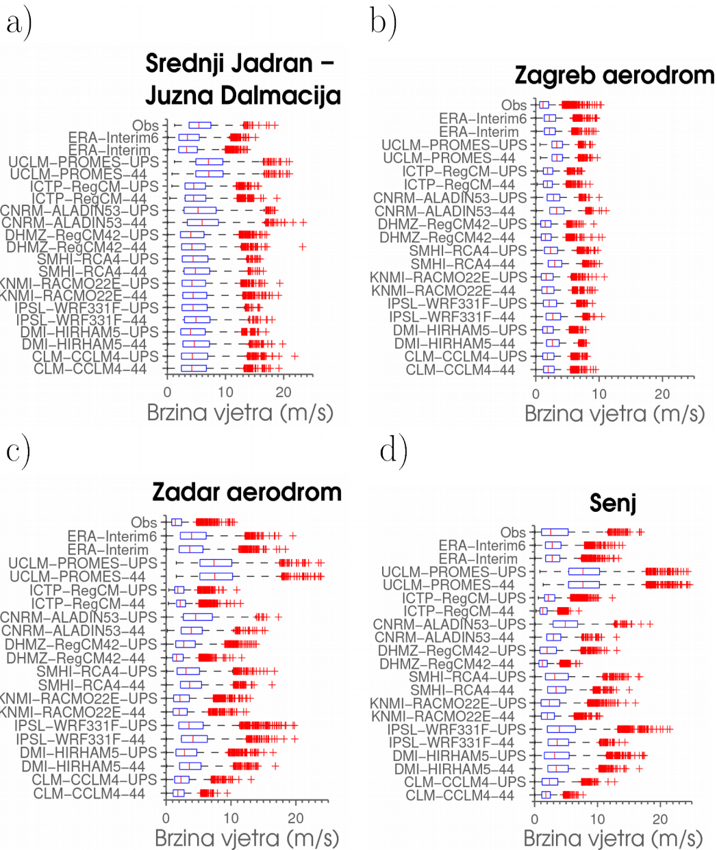
Slika 9. Dijagrami s pravokutnikom brzine vjetrova za simulacije s prostornim korakom 0.44^\circ i UPS simulacije koristeći NN interpolaciju. a) Lokacije nad otvorenim morem (Srednji Jadran - Južna Dalmacija), b) postaja u unutrašnjosti (zračna luka Zagreb), c) obalna postaja u ravničarskom terenu (zračna luka Zadar) i d) obalna postaja u kompleksnom terenu (Senj). Pravokutnik obuhvaća vrijednosti od 25. (P25) do 75. (P75) percentila, crvena linija označava medijan, a crveni križići vrijednosti veće od P75+1.5*(P75-P25) ili manje od P25-1.5*(P75-P25) .
