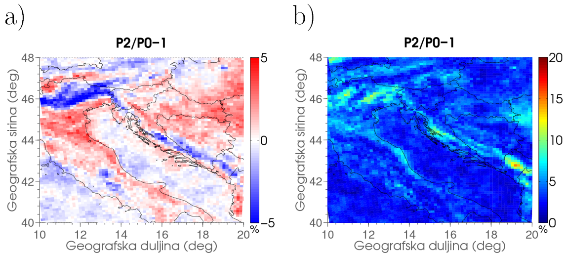
Slika D2. Ansambl medijan (a) i pripadni IQR raspon (b) relativne promjene ( P2/P0-1 ) po simulacijama za 99. percentil brzine vjetrova za RCP8.5 scenarij u zimskoj sezoni. Ansambl se sastoji od devet članova, osim u P3 koji sadrži pet članova na 6-h skali.
