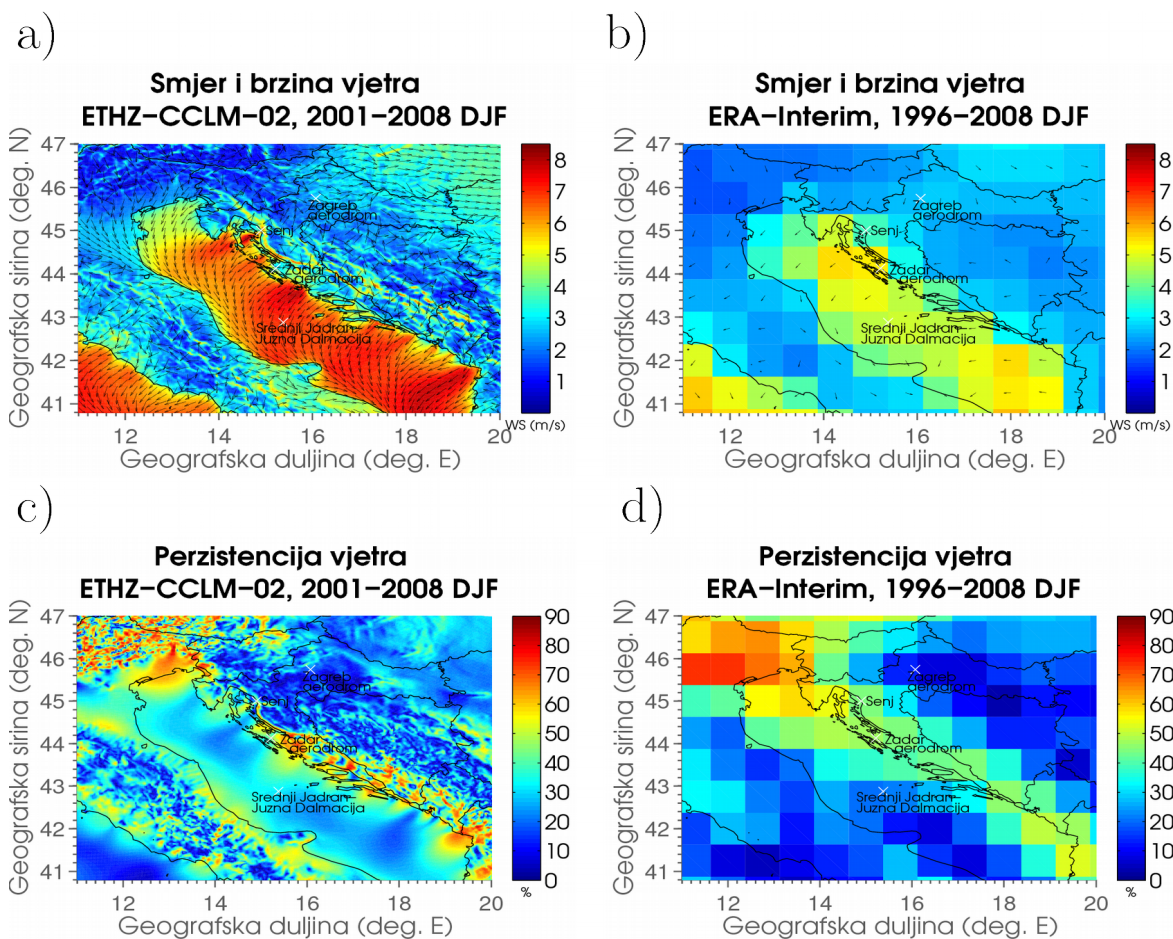
Slika 4. Zimski (DJF) sezonski vektorski srednjaci (označeno vektorima; a, b), srednjaci brzine (označeno bojama; a, b) i stalnosti vjetra (označeno bojama; c, d) nad širim jadranskim područjem iz ERA-Interim reanalize (desno) i ETHZ-CCLM-02 simulacije (lijevo). Vektori vjetra su normalizirani brzinom vjetra i daju informaciju samo o smjeru vjetra. Bijeli simboli predstavljaju postaje koje su detaljno diskutirane u tekstu.
