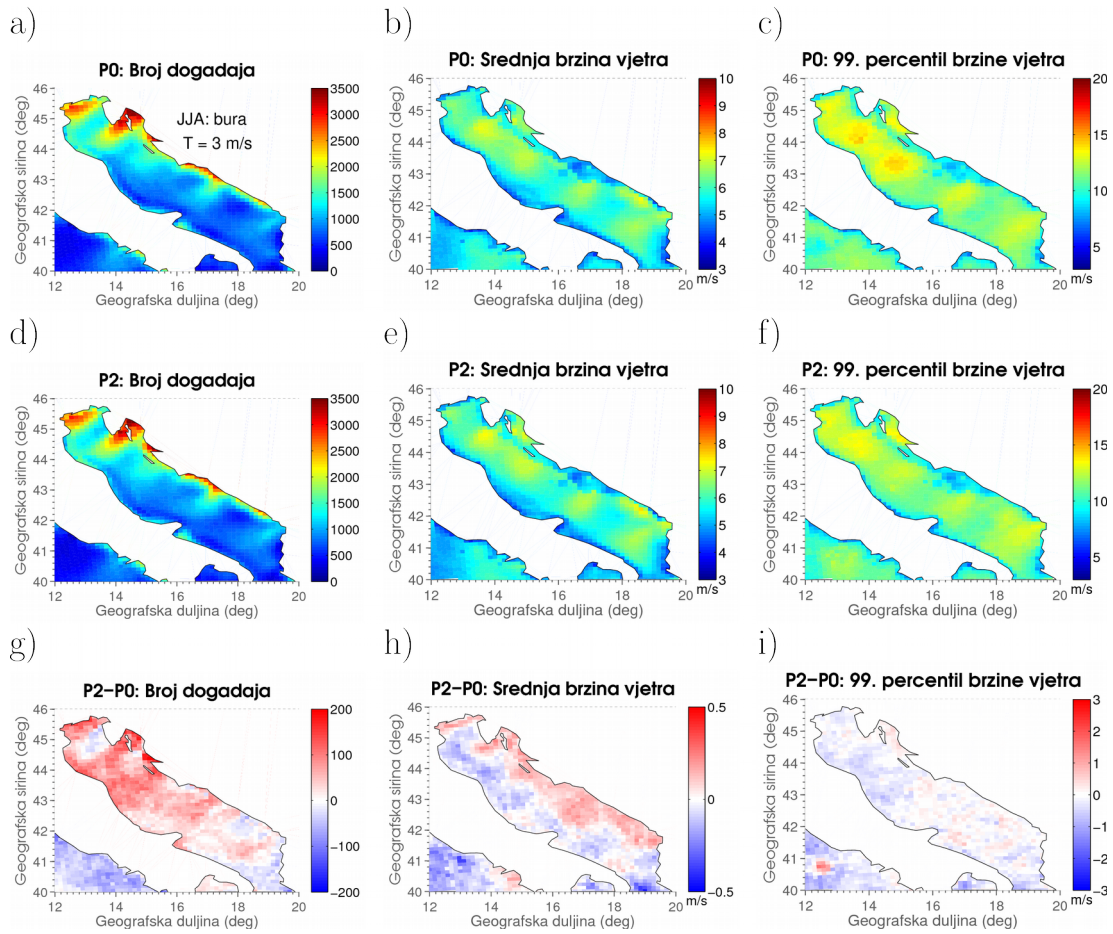
Slika B2. Isto kao Slika B1, ali za JJA sezonu.
