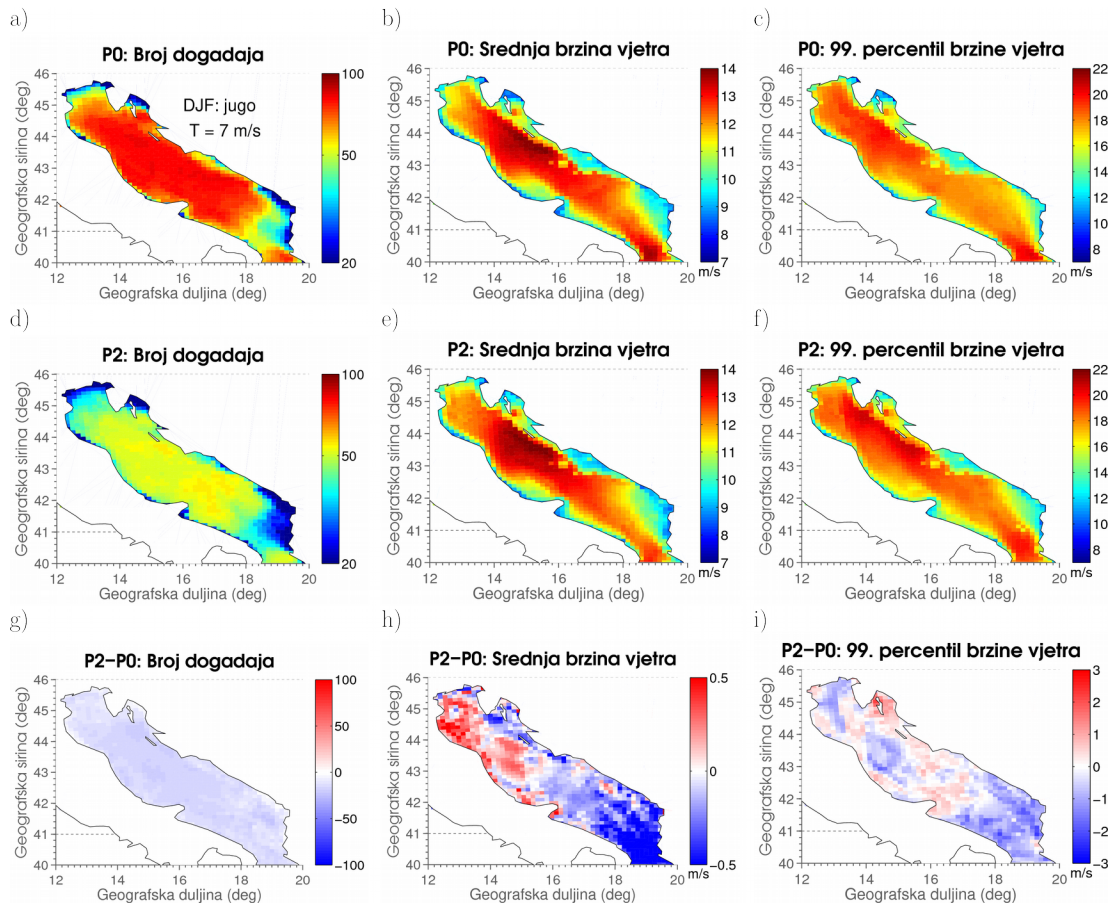
Slika C3. Isto kao Slika C1, ali za jugo (112.5°-157.5°).
