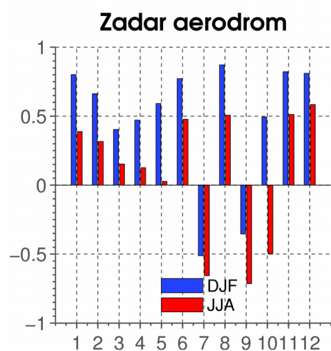
Slika 12. Modificirani BSS brzine vjetra (na y - osi) izračunat je koristeći ERA-Interim simulaciju za zimsku (DJF) i ljetnu (JJA) sezonu za 0.11^\circ i 0.02^\circ NN simulacije. Prikaz za obalnu postaju u ravničarskom terenu (zračna luka Zadar). Svaki broj na x - predstavlja jedan model naznačen u Tablici 1.
