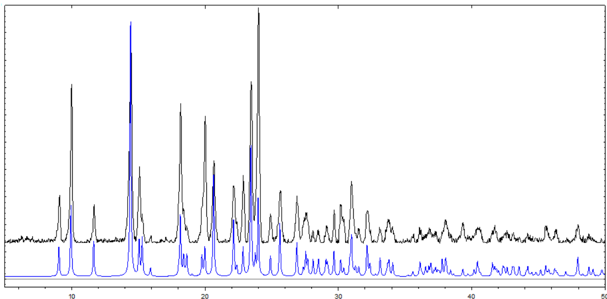
Slika D38. Difraktogram praha [\text{Ni}(\text{acac})_2(\text{Ipz})_2] ( 16b ) (crno), računati (plavo).
