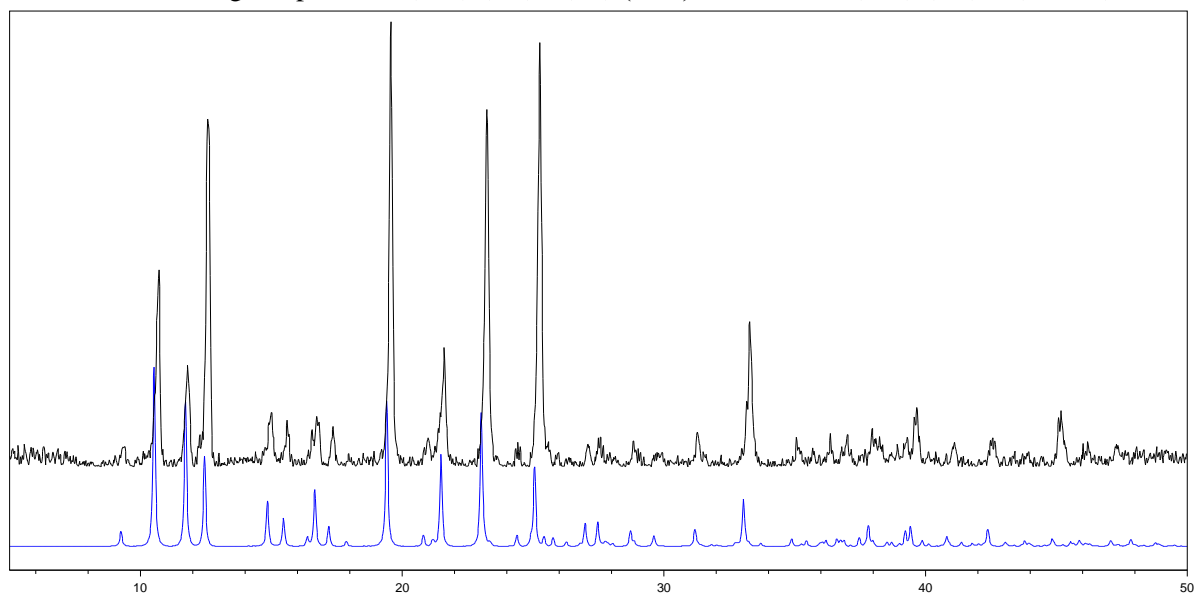
Slika D23. Difraktogram praha [Co(tfac) 2 (isn) 2 ] ( 8a ) (crno), računati (plavo).
