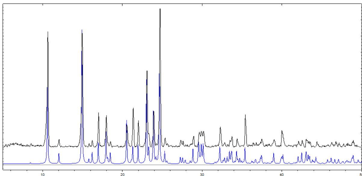
Slika D39. Difraktogram praha [\text{Co}(\text{acac})_2(5\text{-Brpm})_2] ( 17a ) (crno), računati (plavo).
