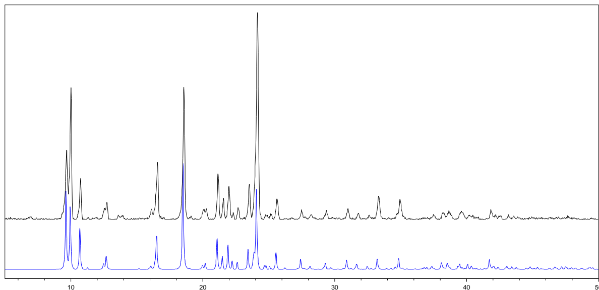
Slika D14. Difraktogram praha [\text{Co}(\text{hfac})_2(\text{qz4on})_2] ( 4a ) (crno), računati (plavo).
