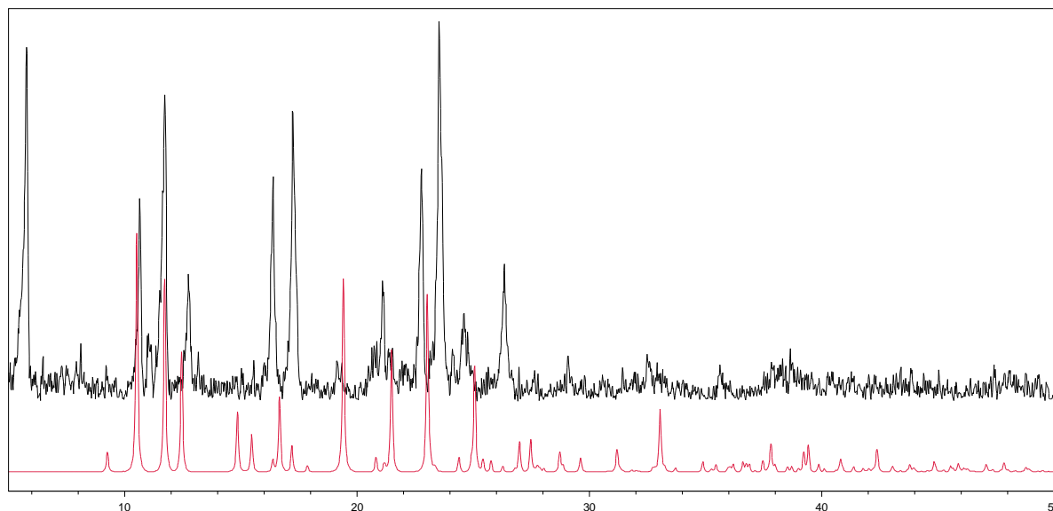
Slika D24. Difraktogram praha [Ni(tfac) 2 (isn) 2 ] ( 8b ) (crno), računati [Co(tfac) 2 (isn) 2 ] (crveno).
