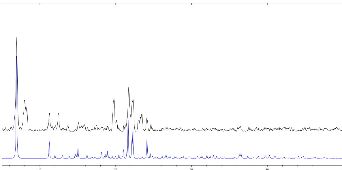
Slika D25. Difraktogram praha [Co(hfac) 2 (nia) 2 ] ( 9a ) (crno), računati (plavo).
