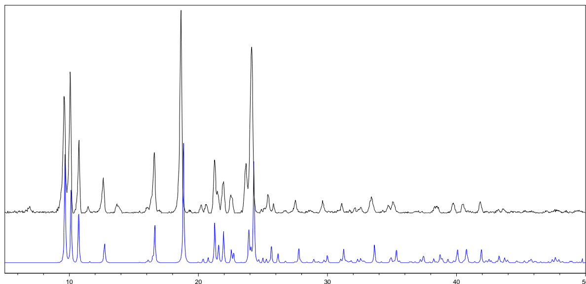
Slika D15. Difraktogram praha [\text{Ni}(\text{hfac})_2(\text{qz4on})_2] ( 4b ) (crno), računati (plavo).
