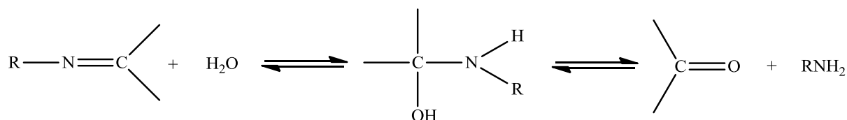
Slika 2.3. Hidroliza dvostruke \text{C}=\text{N} - veze.
