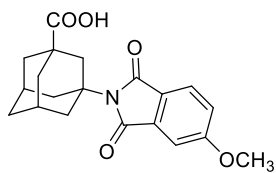
Prilog 35. ^1\text{H} (DMSO- d_6 , 300 MHz) i ^{13}\text{C} (DMSO- d_6 , 150 MHz) NMR spektri spoja 9 .
