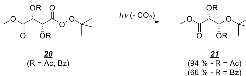
Shema 10. Sinteza kiralnih acikličkih acetala 21 fotodekarboksilacijom peroksitartarata 20 . 47
