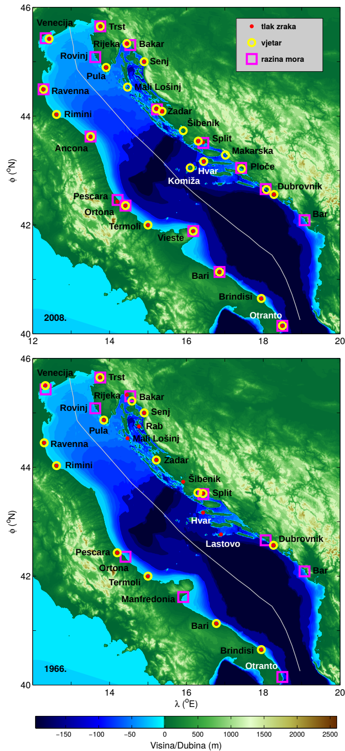
Slika 2.3: Batimetrija Jadrana, lokalna orografija i lokacije mareografskih i meteoroloških postaja čiji podaci su korišteni za analizu poplave iz 2008. ( gore ) i 1966. ( dolje ). Dubine veće od 250 m prikazane su istom bojom. Također je prikazan profil duž bazena korišten na slici 2.9.
