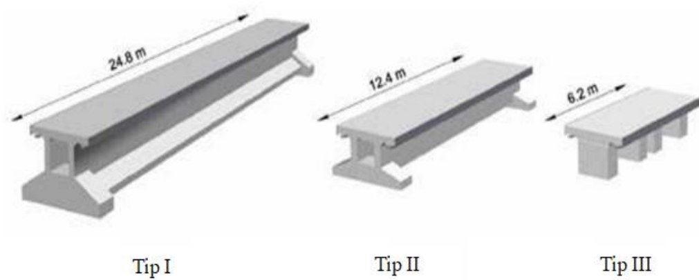
Slika 7. Standardni tipovi nosača Maglev sustava
