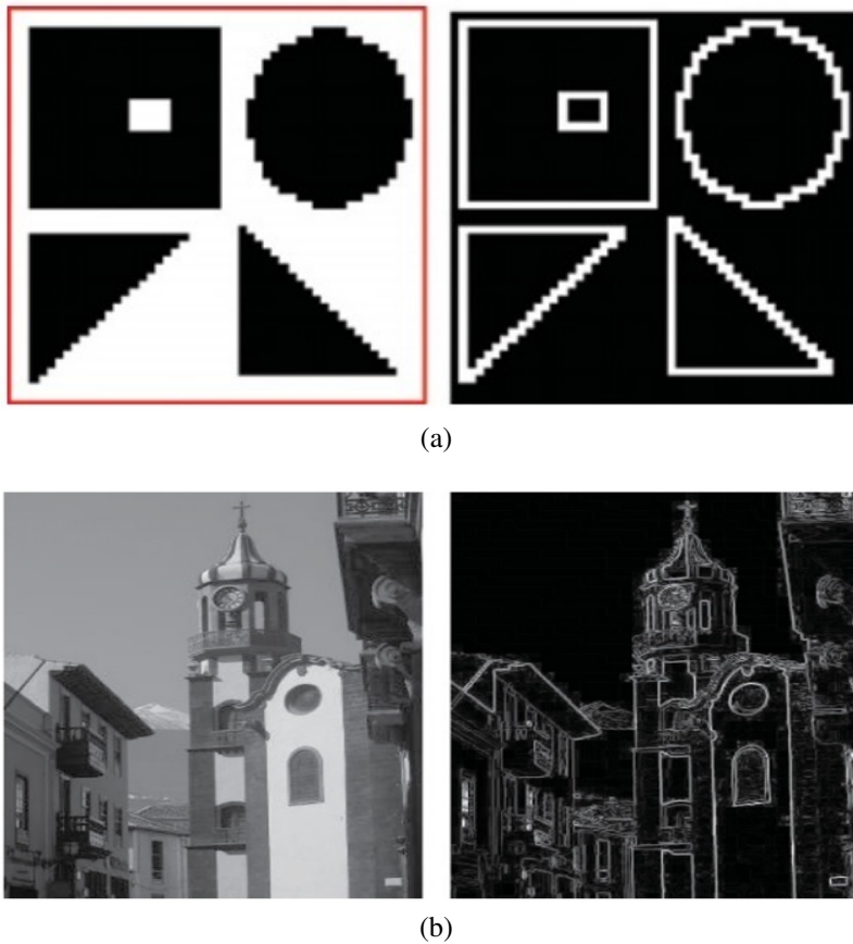
Slika 4.8: Prikaz djelovanja Robertovog detektora rubova na binarnoj slici (a) i sivoj slici (b).
