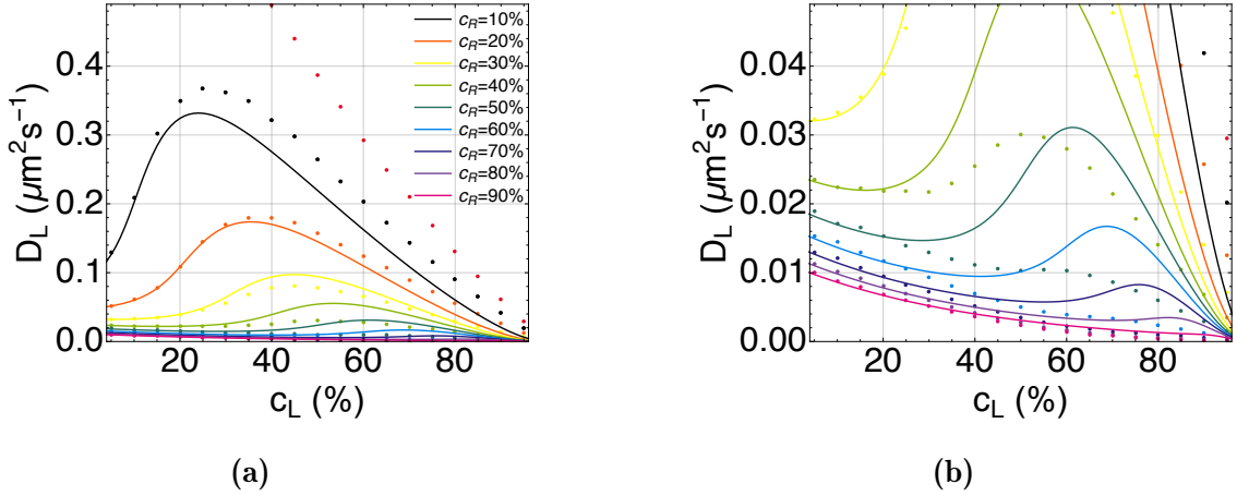
Slika 4.7: Usporedba simulacijskih rezultata i teorijske procjene efektivnih difuzijskih koeficijenata prema izrazu (2.19). Graf (b) je uvećanje grafa (a) po y -osi, s legendom identičnom grafu (a) . Simulacijski rezultati su prikazni točkama, a analitička procjena punim linijama. Crvene točke na grafu (a) i (b) predstavljaju simulaciju slobodne difuzije liganada.
