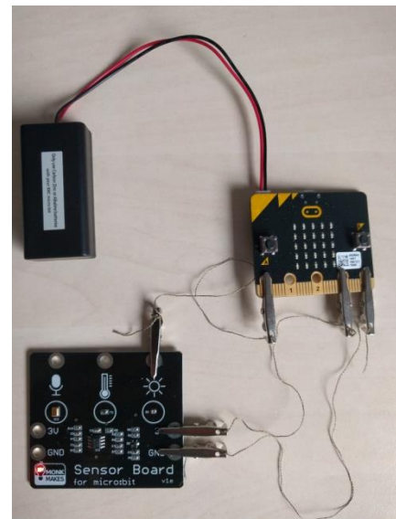
Slika 19. Poslije spajanja
