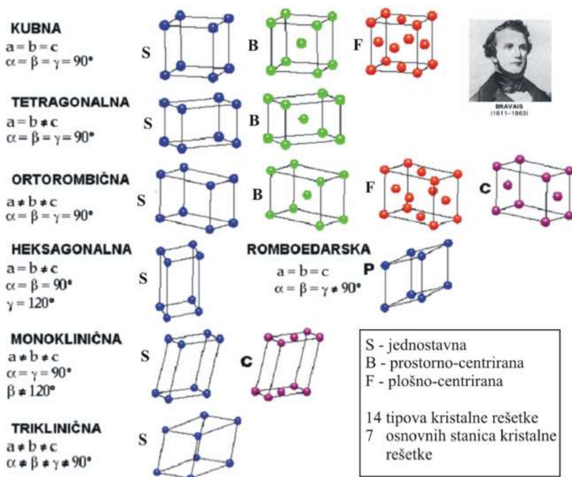
Slika 17 - Bravaisova podjela kristalnih rešetki
