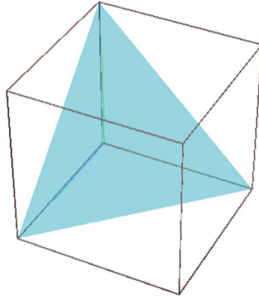
Slika 47 – ravnina \Pi zapisana Millerovom notacijom (111)
