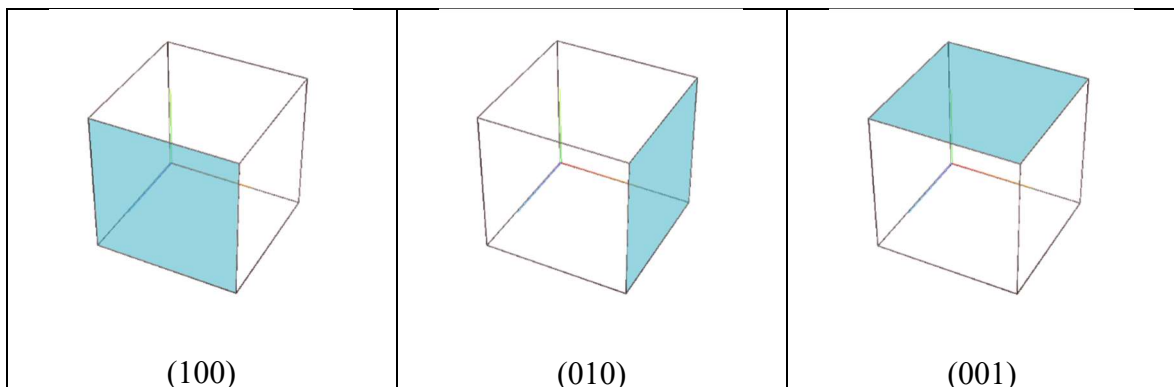
Tablica 5 - primjeri ravnina zapisani Millerovom notacijom
