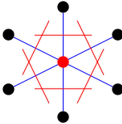
Slika 11 - Wigner-Seitzova ćelija
