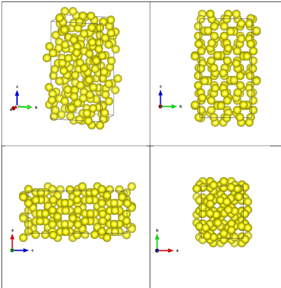
Tablica 2 - prikaz 3D modela molekule sumpora na temperaturi 298K gledano iz različitih smjerova
