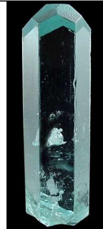
Slika 39 - kristal berila (verzija "Aquamarine") 13
