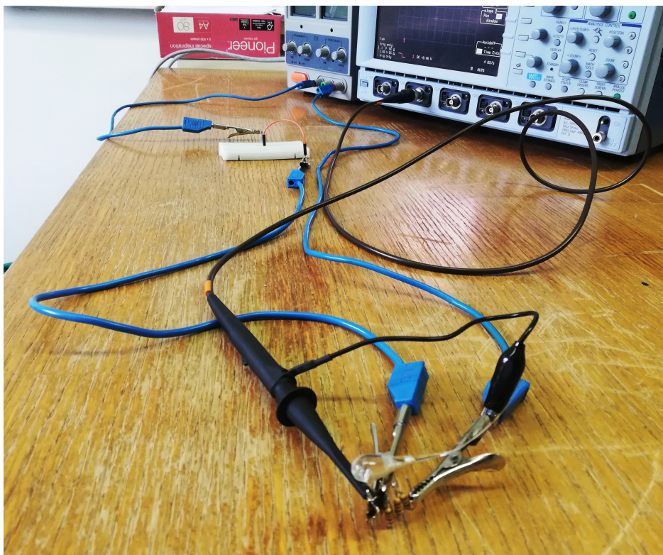
Slika 3.7: Postav za mjerenje brzine u Rupertovoj kaplji.
