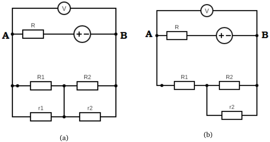
Slika 3.4: Strujni krug za mjerenje brzine eksplozije prije (a) i tokom (b) eksplozije.
