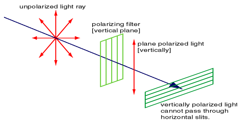
Slika 2.3: Polarizacija svjetlosti.
