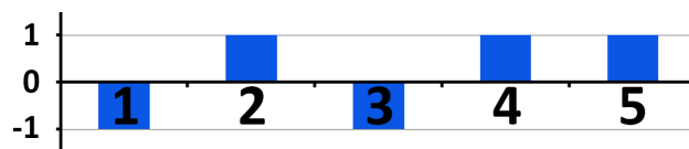
Slika 3.5: Paulov vektor poteza
