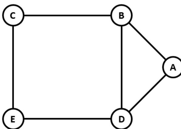
Slika 3.1: Neusmjereni graf
