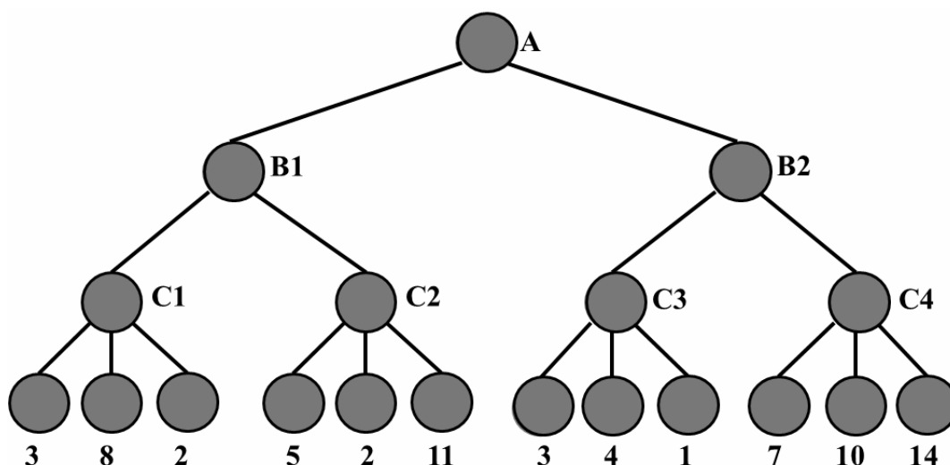
Slika 4.2: Minimax stablo
