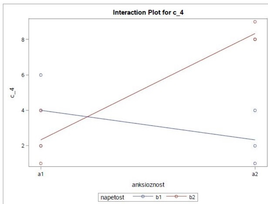
Slika 3.4: Interakcijski graf za zavisnu varijablu c_4 po grupnim varijablama anksioznost i napetost-Ispis iz SAS-a
