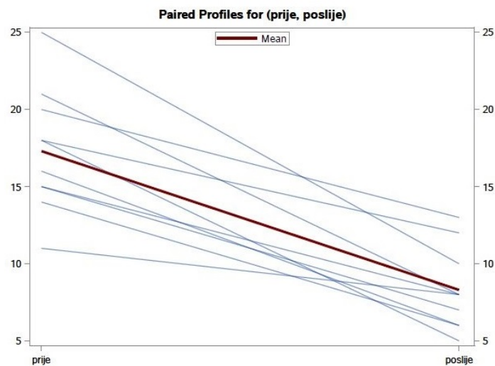
Slika 1.2: Grafički prikaz razlike "prije-poslije"-Ispis iz SAS-a
