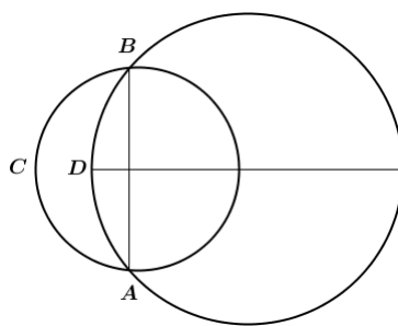
Slika 3.5: Mjesec
