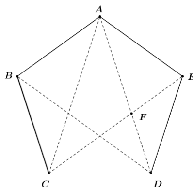
Slika 2.15: Konstrukcija peterokuta
