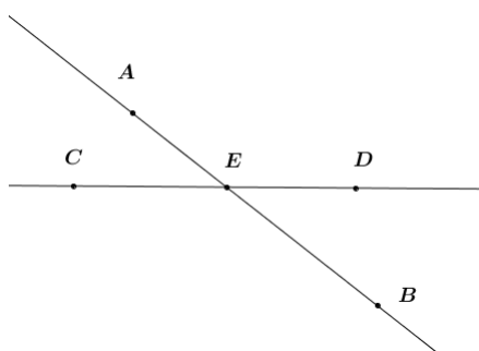
Slika 1.1: Vršni kutovi
