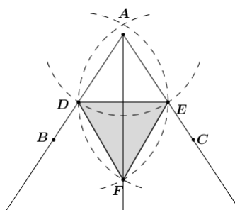
Slika 3.11: Bisekcija kuta
