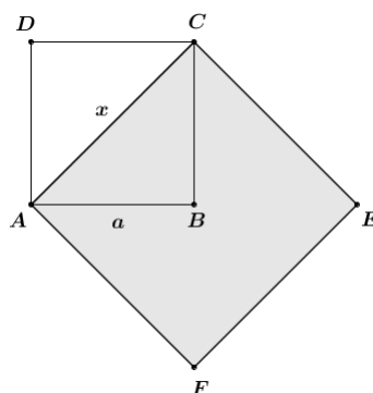
Slika 3.15: Udvostručenje kvadrata
