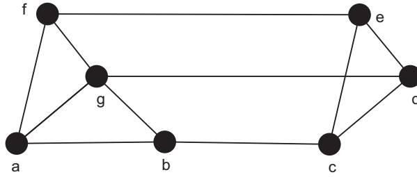
Slika 44: Matroid ranga 4.
