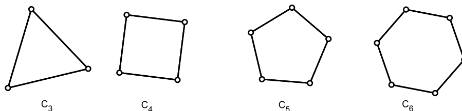
Slika 13: Ciklusi.
