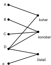
Slika 22: Bipartitni graf.
