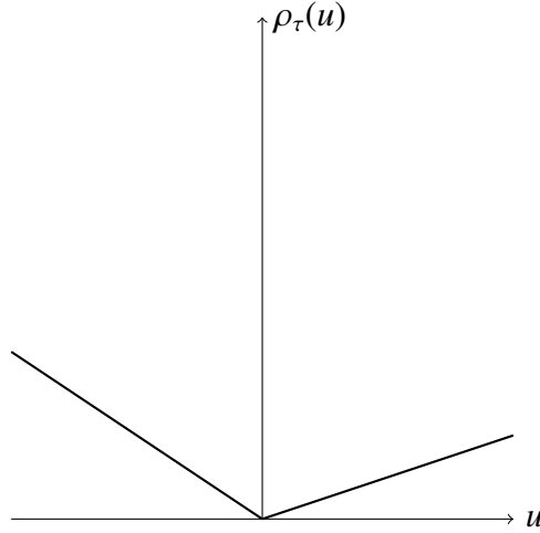
Slika 1.2: Funkcija gubitka
