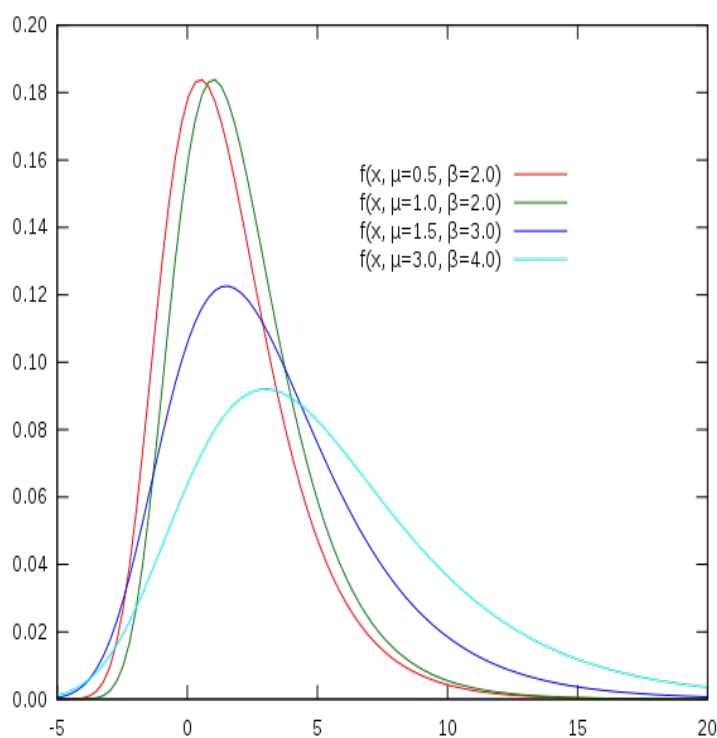
Slika 1.1: Funkcija gustoće
