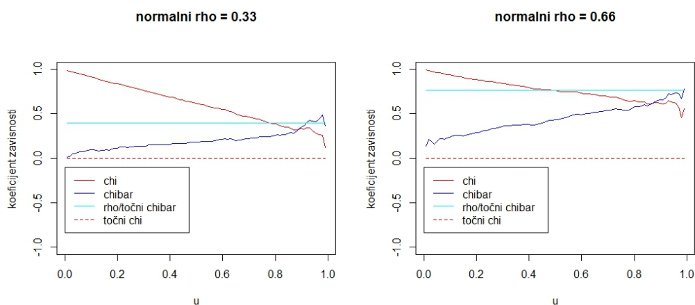
Slika 3.3: Grafovi \chi(u) i \bar{\chi}(u) za generirane normalne podatke
