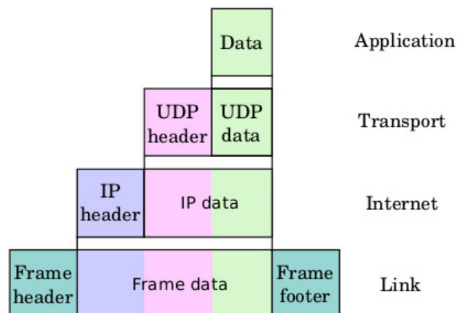
Slika 2.2: Primjer enkapsulacije u datagram po slojevima TCP/IP stoga.
