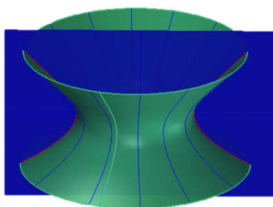
Slika 1.7: Meridijani
