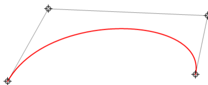
Slika 2.3: Bézierova krivulja 3. stupnja
