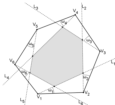
Slika 2.5: Presjek \mathcal{P}^-(\theta)
