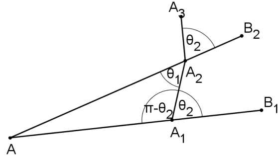
Slika 2.9: Trokut AA_1A_2
