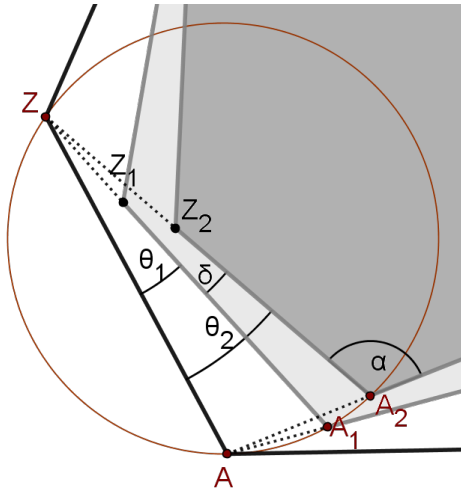
Slika 2.8: Koncikličke točke
