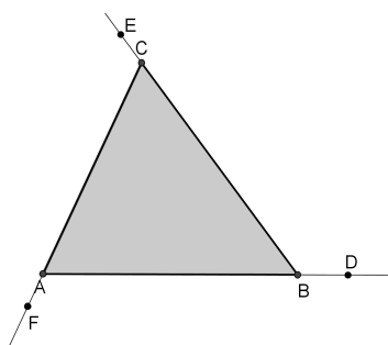
Slika 1.7: \theta = 0^\circ
