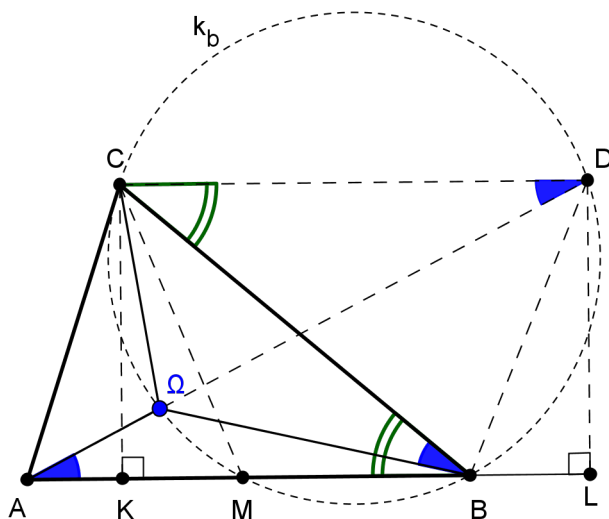
Slika 1.11: Dokaz teorema 1.2.2
