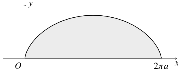
Slika 3.8. Površina ispod svoda cikloide.
