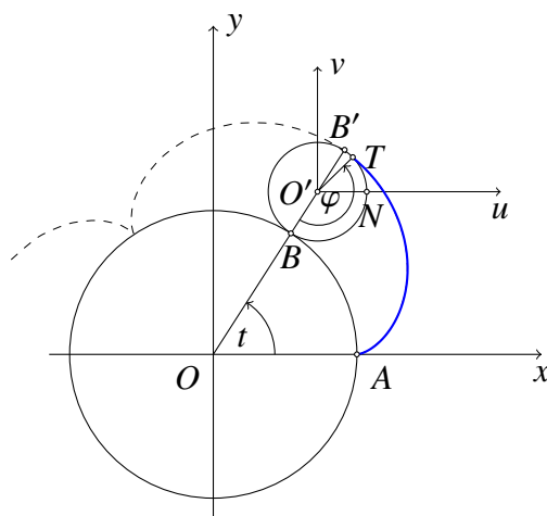
Slika 3.9. Uz izvod parametarskih jednadžbi epicikloide.
